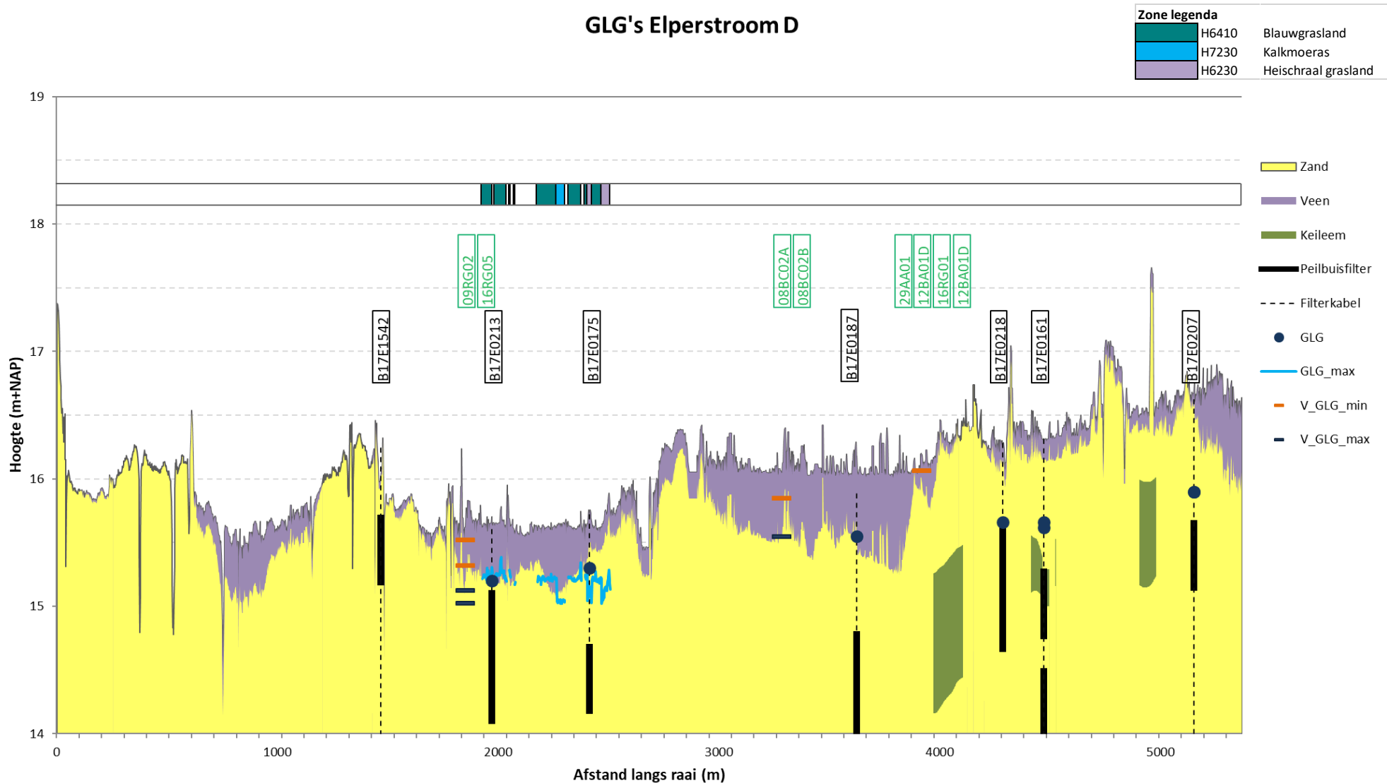
Figuur 5-4 Resultaten van de toetsing van de actuele GLG en optimale GLG, raai D Zuid-Noord beekdal
