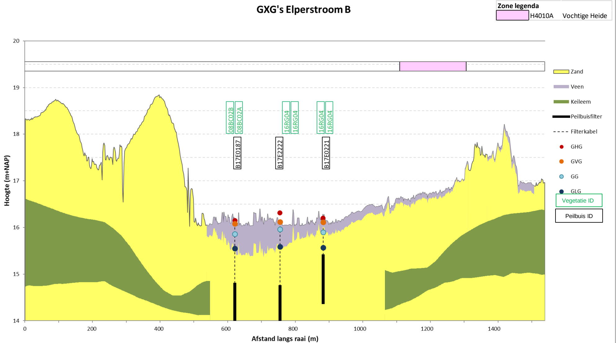
Figuur 2-18 GxG's ondiepe filters, raai B West-oost door Oosterma
