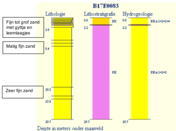
Figuur 2-4. twee boringen in deelgebied Reitma
