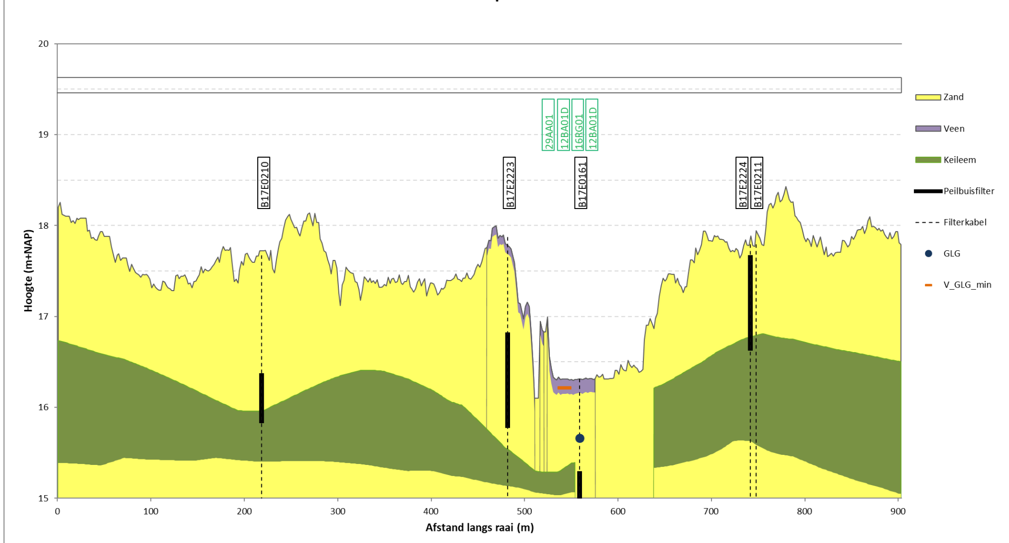
Figuur 5-3. Resultaten van de toetsing van de actuele GLG en optimale GLG, raai C Stroetma
