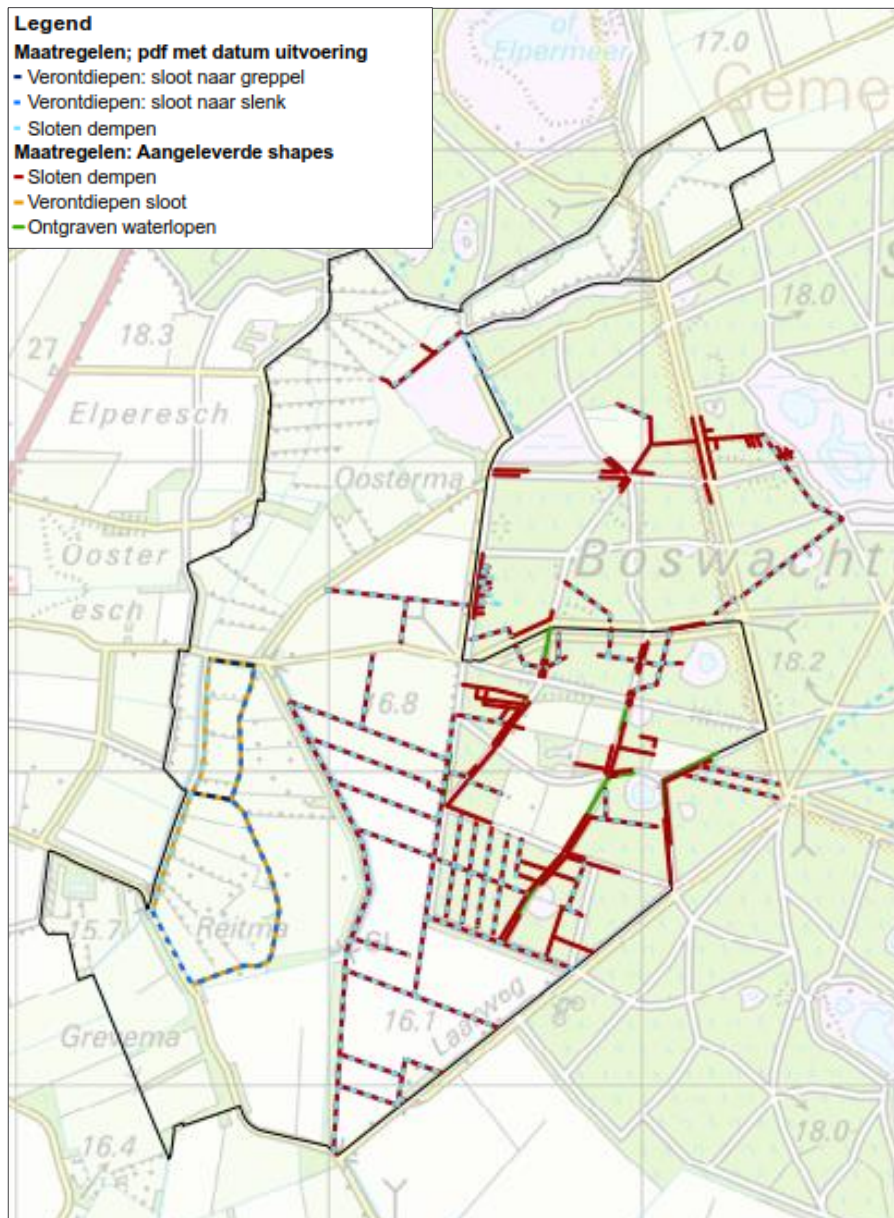
Figuur 3-1 Maatregelenkaart
