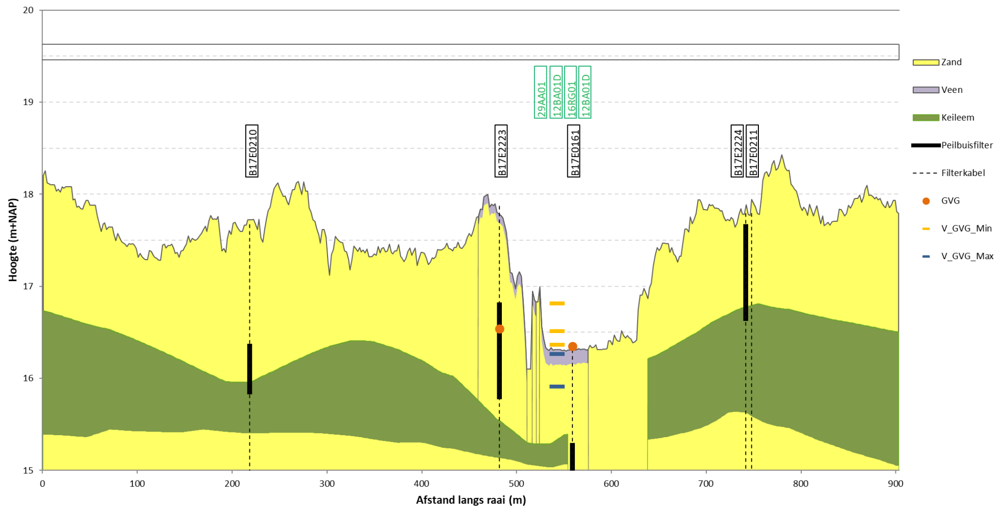
Figuur 5-7 Resultaten van de toetsing van de actuele GVG en optimale GVG, raai C
