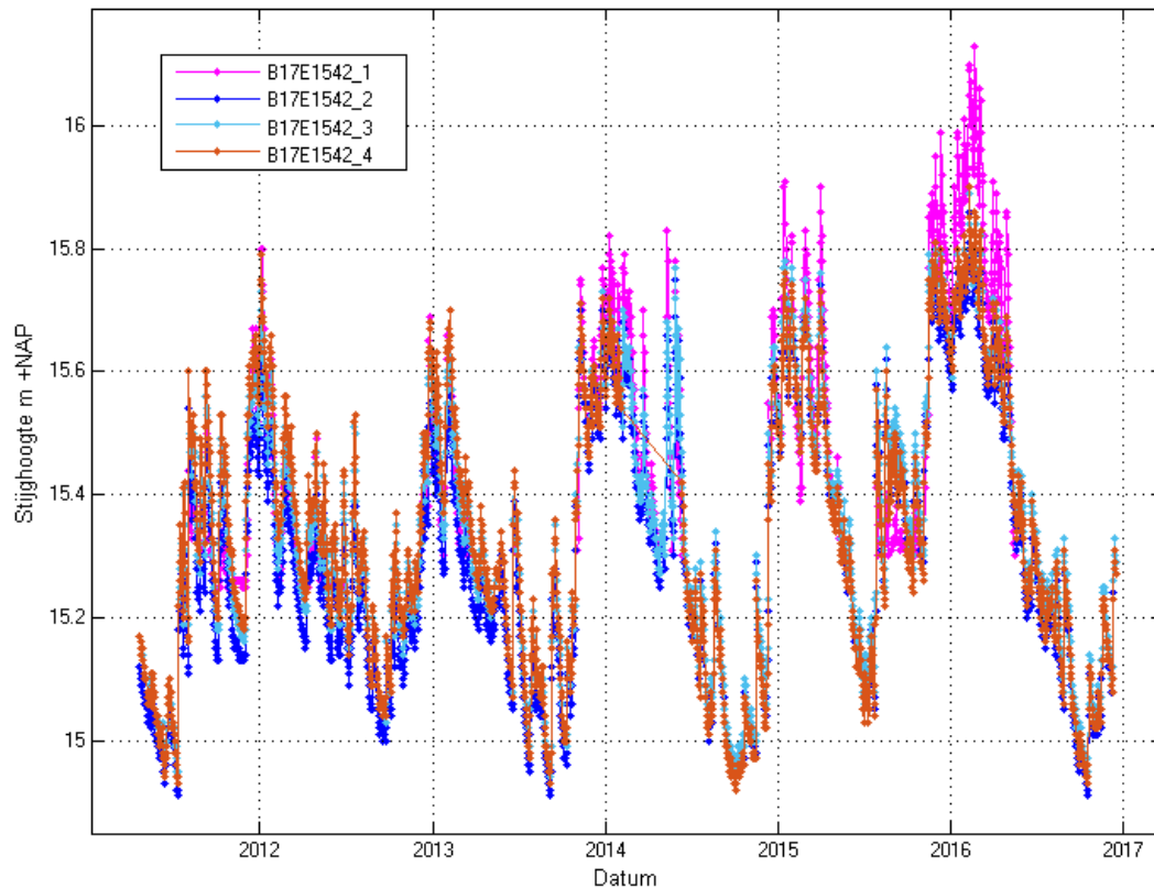
Figuur 5-12. Stijghoogten B17E1542 in deelgebied Grevema
