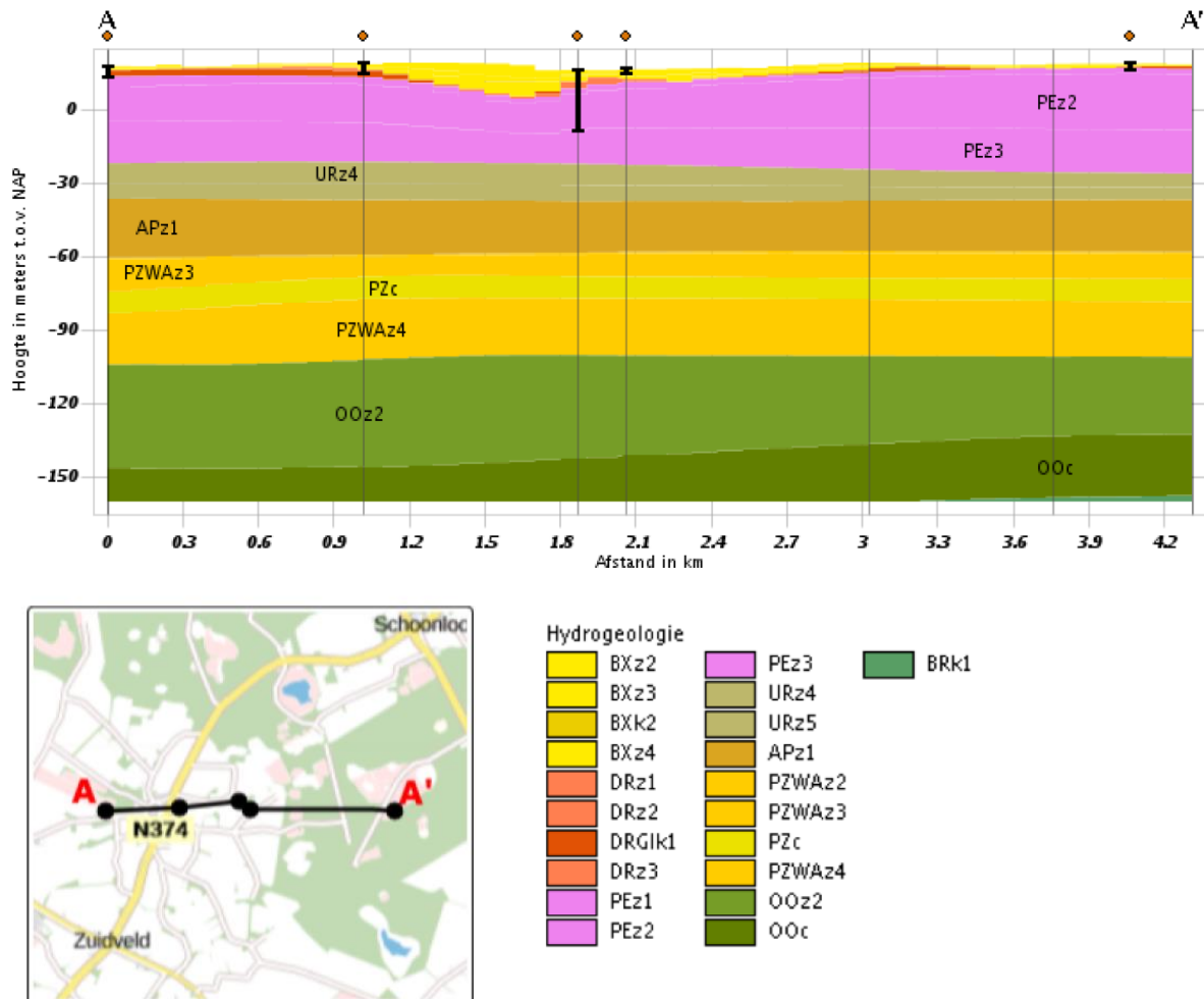
Figuur 2-3 West-Oost dwarsprofiel Elperstroom uit REGIS II.2.
