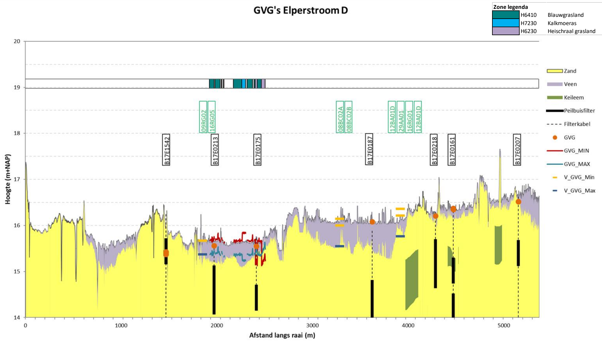
Figuur 5-8 Resultaten van de toetsing van de actuele GVG en optimale GVG, raai D
