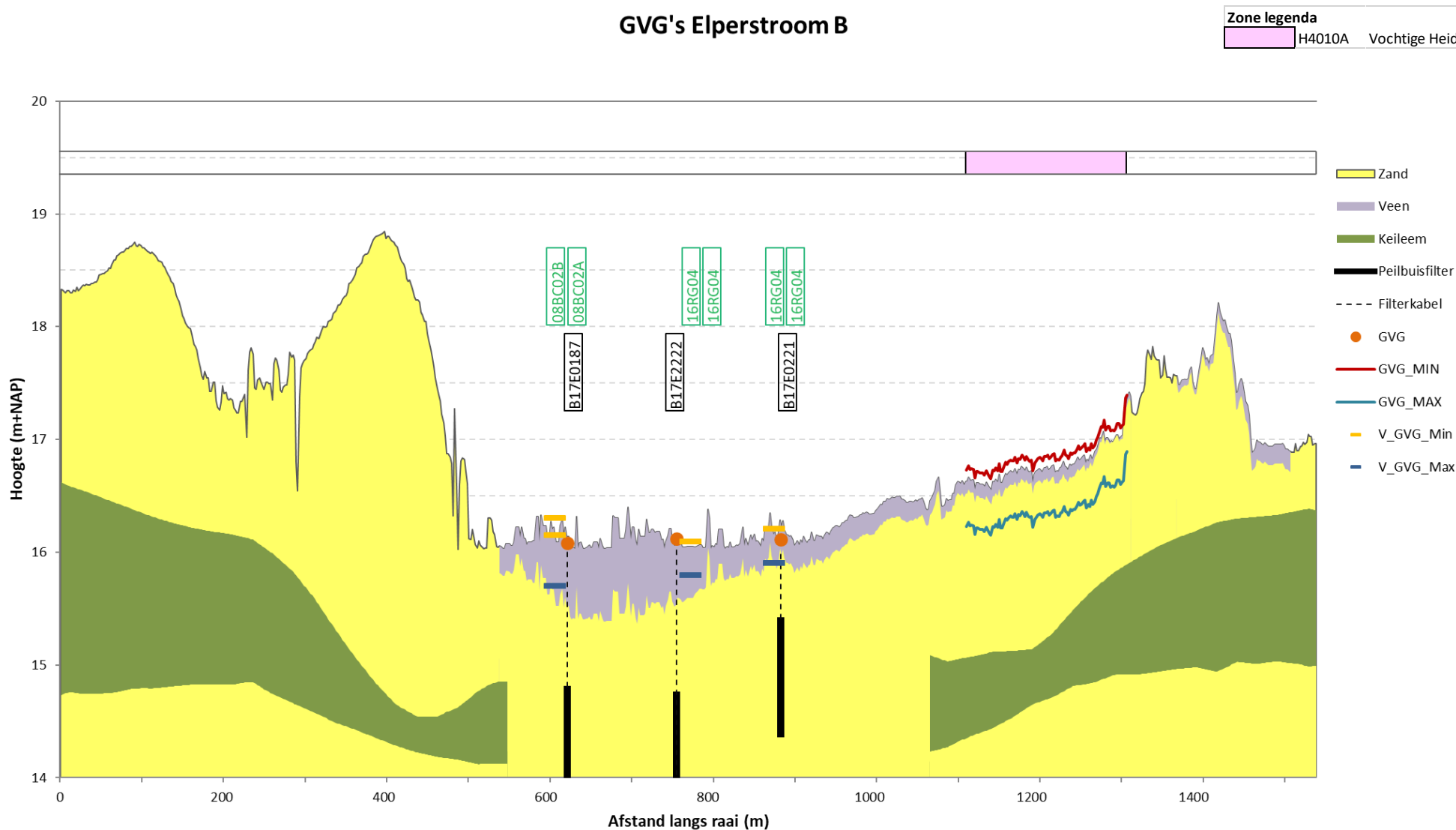
Figuur 5-6 Resultaten van de toetsing van de actuele GVG en optimale GVG, raai B
