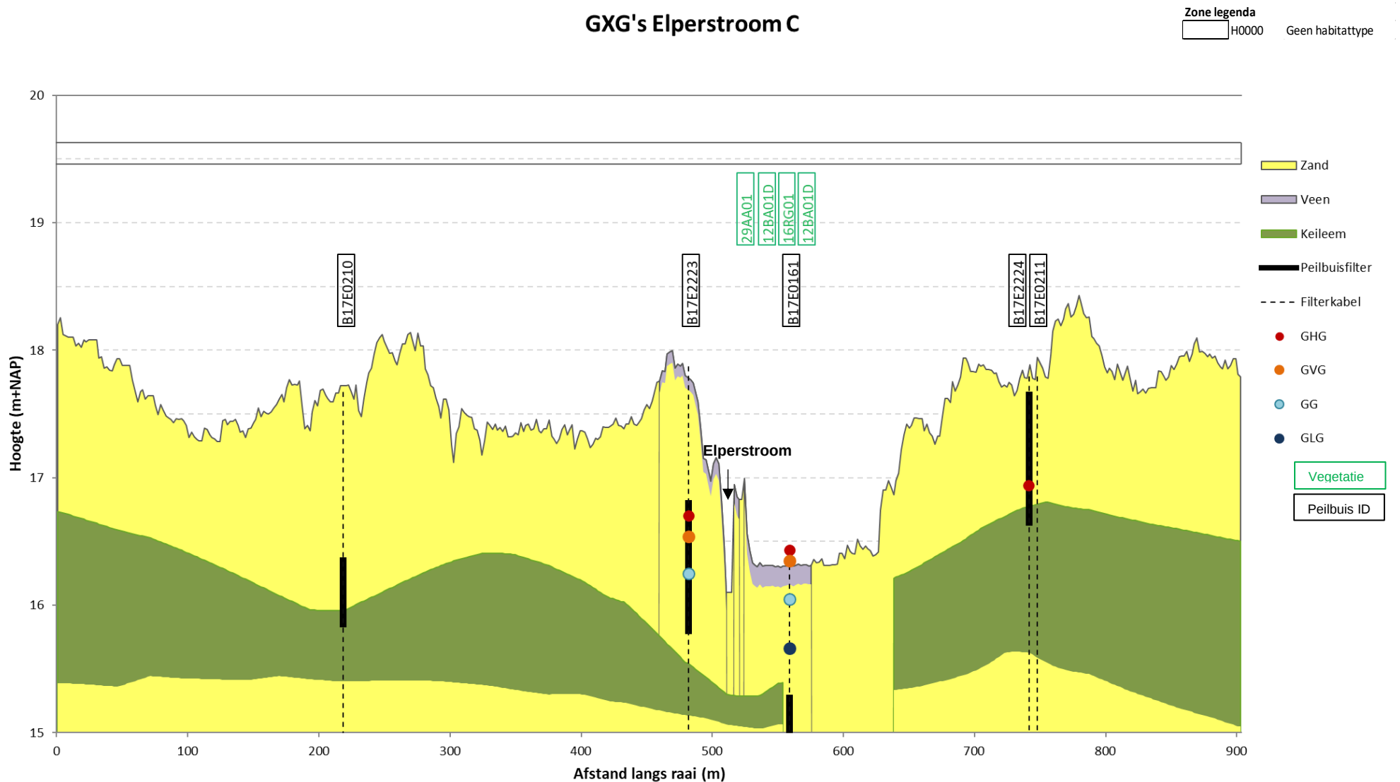
Figuur 2-19. GxG's ondiepe filters, raai C. Noordwest-Zuidoost door Stroetma
