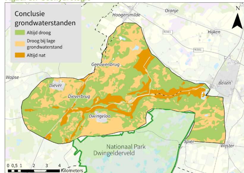
Figuur 3.7 Geohydrologie
