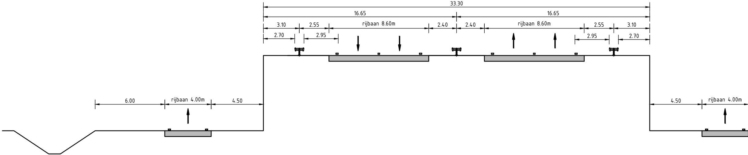
Regionale stroomweg type II (2x2) (Fly-over Knoopunt Gieten) Aardebaan - Maatvoering Provincie Drenthe & CROW
