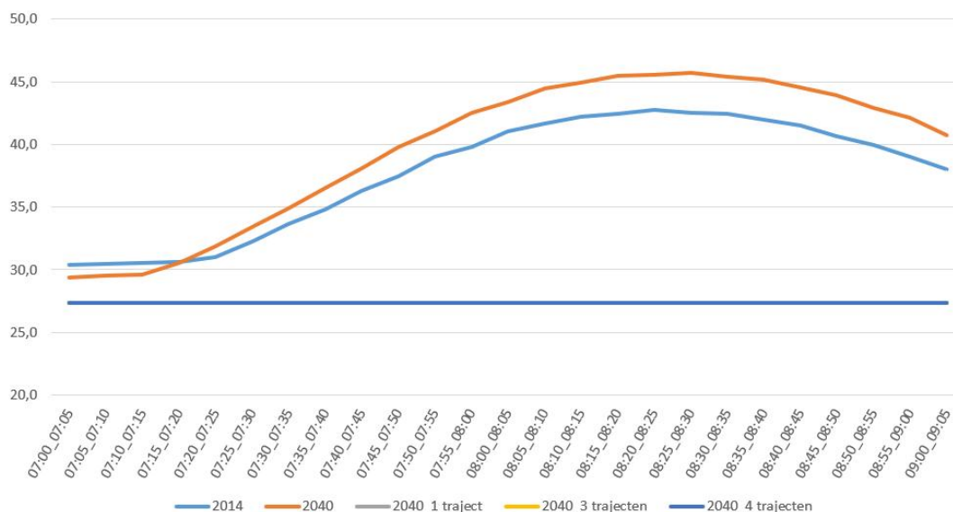
Figuur 4.1 Effecten op gemiddelde rijtijd op totale traject N34 richting noord in ochtendpits
