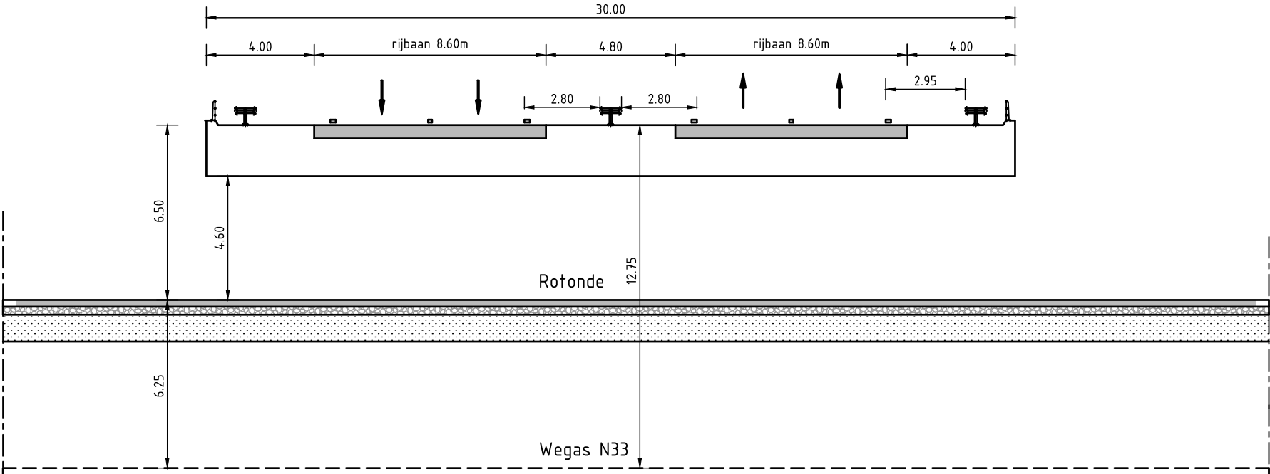
Regionale stroomweg type II (2x2) (Fly-over Knoopunt Gieten) - Maatvoering Provincie Drenthe & CROW
