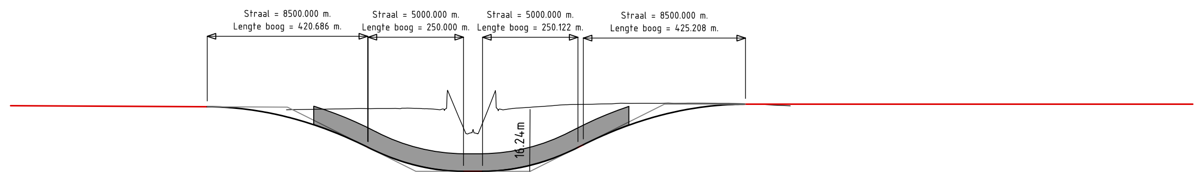
FUNCTIONEEL ONTWERP DIVE-UNDER KNOOPPUNT GIETEN
