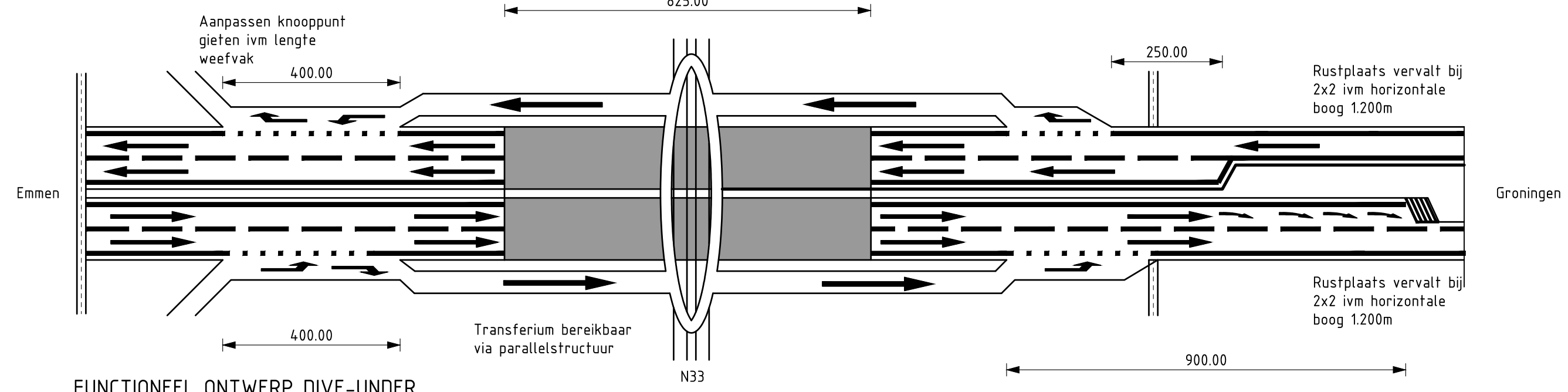
FUNCTIONEEL ONTWERP DIVE-UNDER KNOOPPUNT GIETEN
