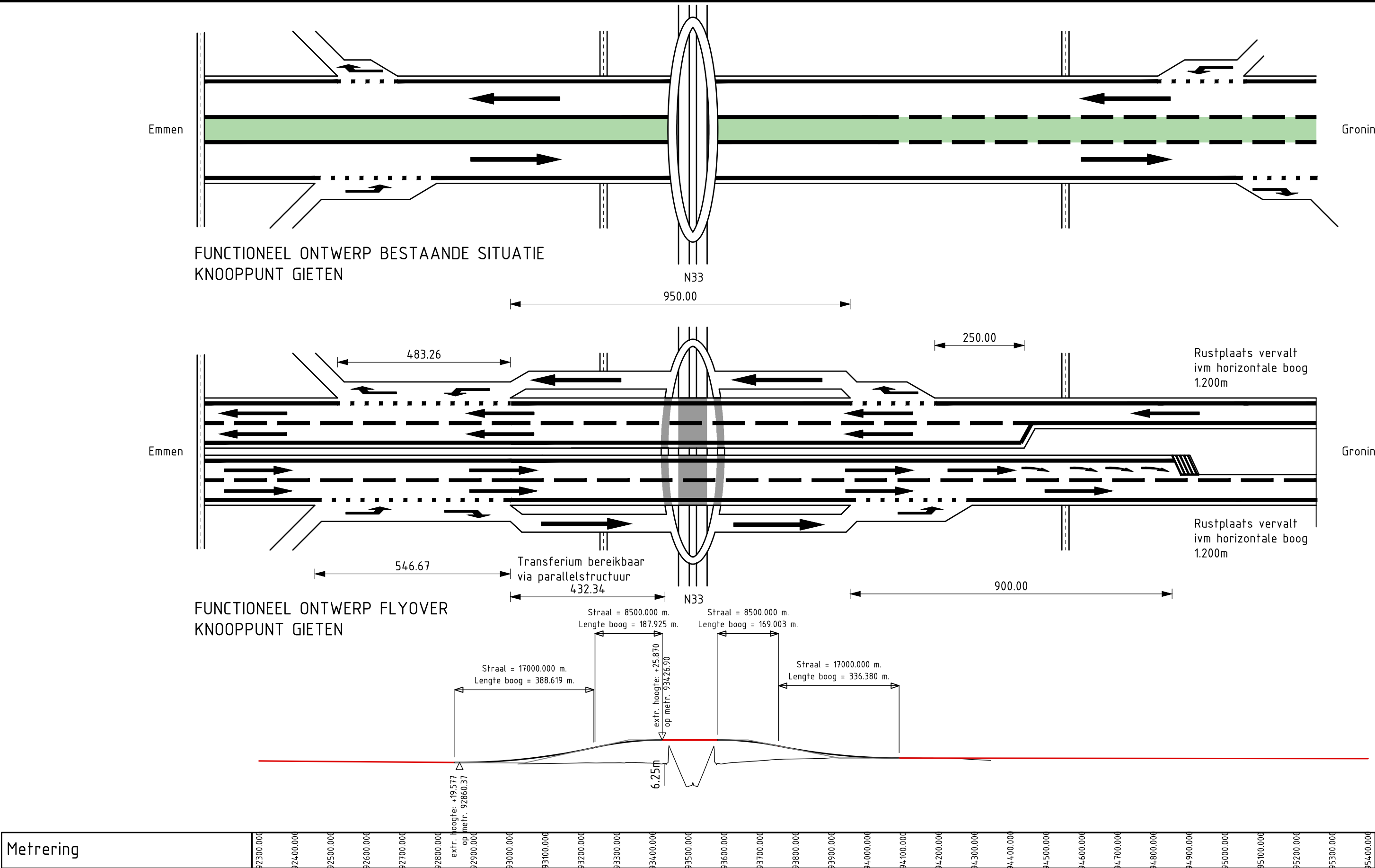
LENGTEPROFIEL FLYOVER
