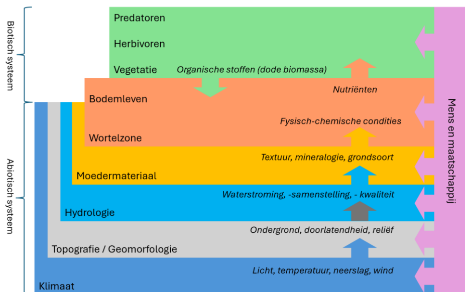
Figuur 1: Rangordemodel van de samenhang van biotische en abiotische onderdelen van de landschapsecologie. Ieder gekleurd vak geeft een component van het systeem weer. Per component zijn de bepalende processen weergegeven. De pijlen geven de dominante beïnvloeding weer. De standplaatsfactoren worden bepaald door de fysisch-chemische condities en de nutriënten. Figuur is aangepast naar figuur 1.4 uit Stobbelaar et al 2022.
