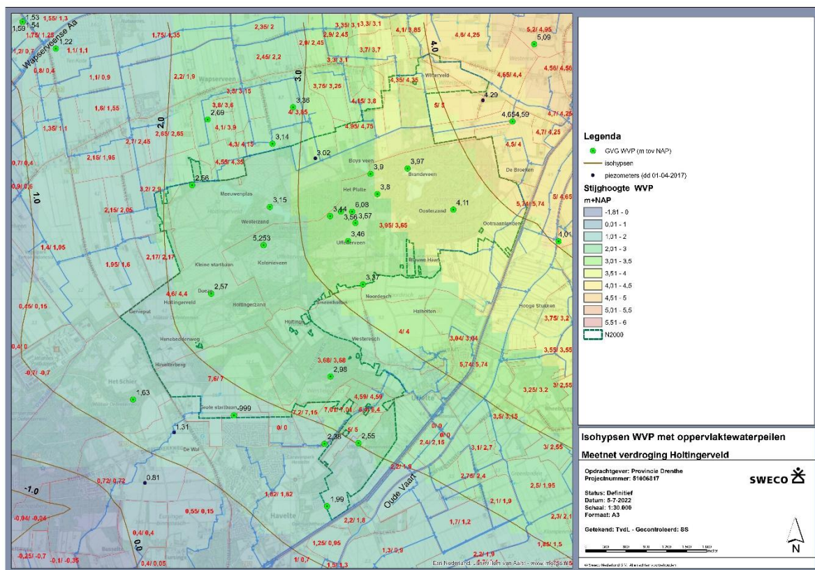
Figuur 2.9 Isohyphen van het eerste watervoerende pakket onder het keileem (overgenomen uit Van der Linden, 2022).
