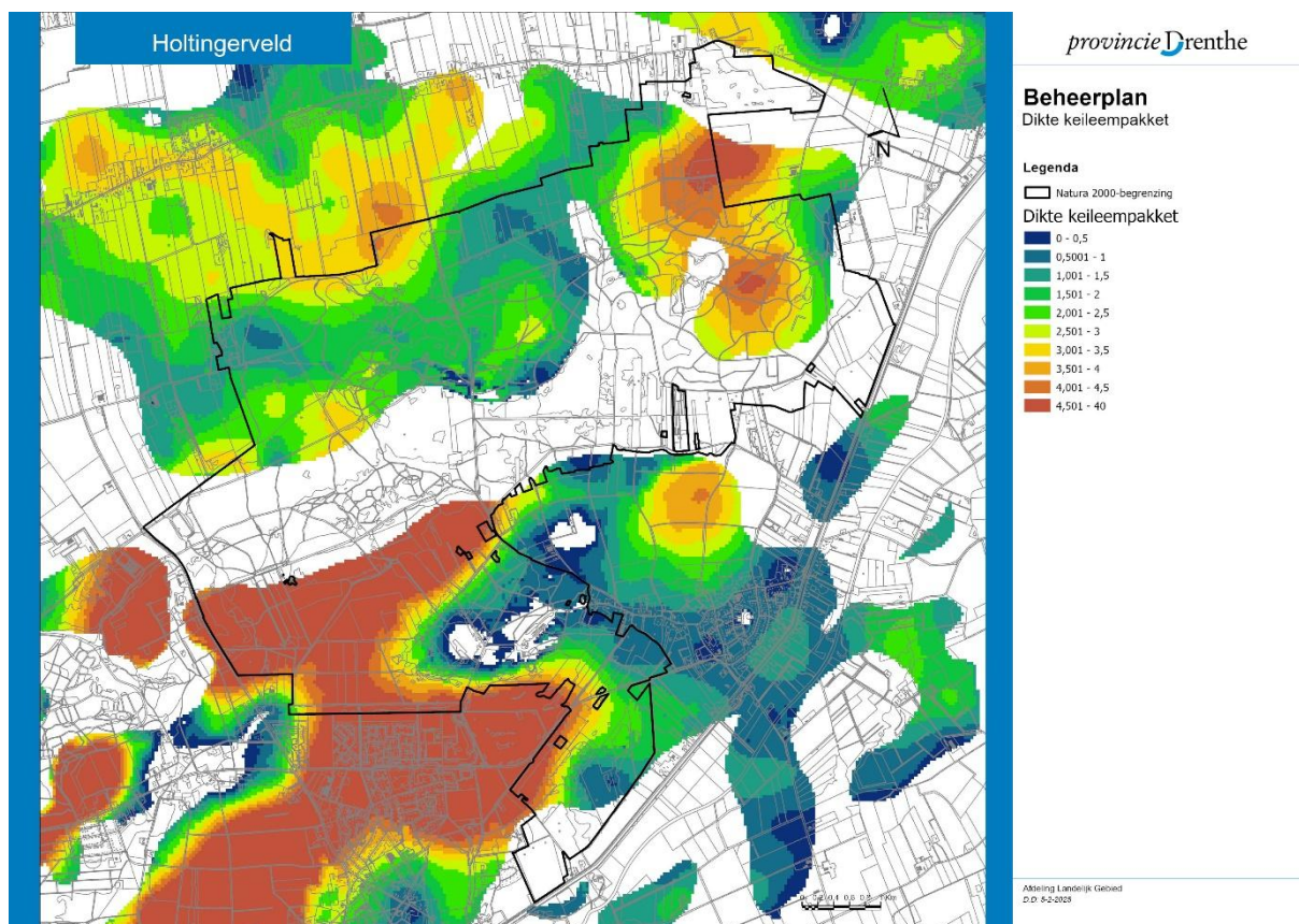
Figuur 2.7: dikte van het keileem
