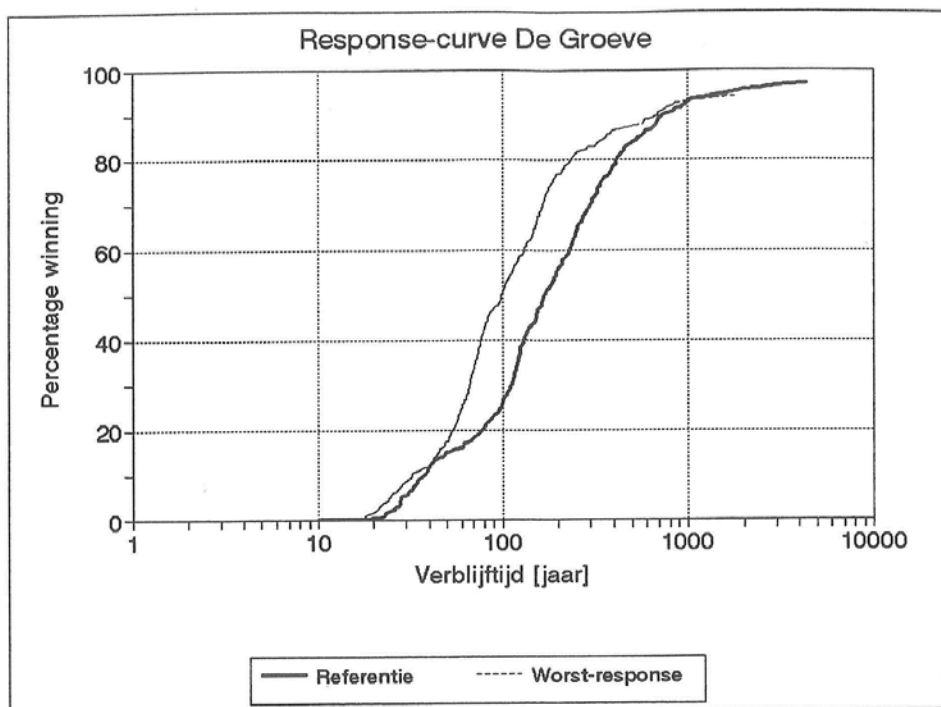
Figuur 4-4 Responsecurve De Groeve (IWACO, 1993)
