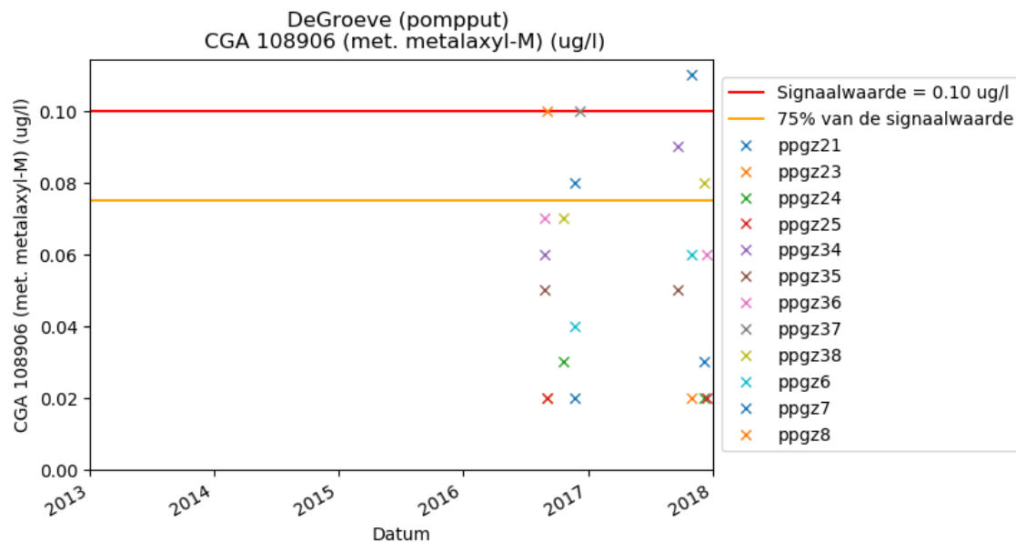
Figuur 5-2 Ontwikkeling metaboliet metalaxyl-M pompputten
