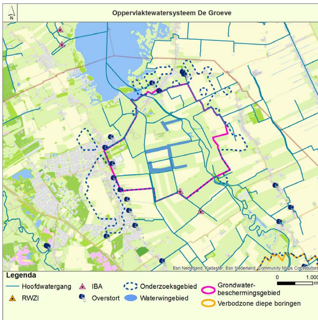
Figuur 6-4 Oppervlaktewatersysteem De Groeve
