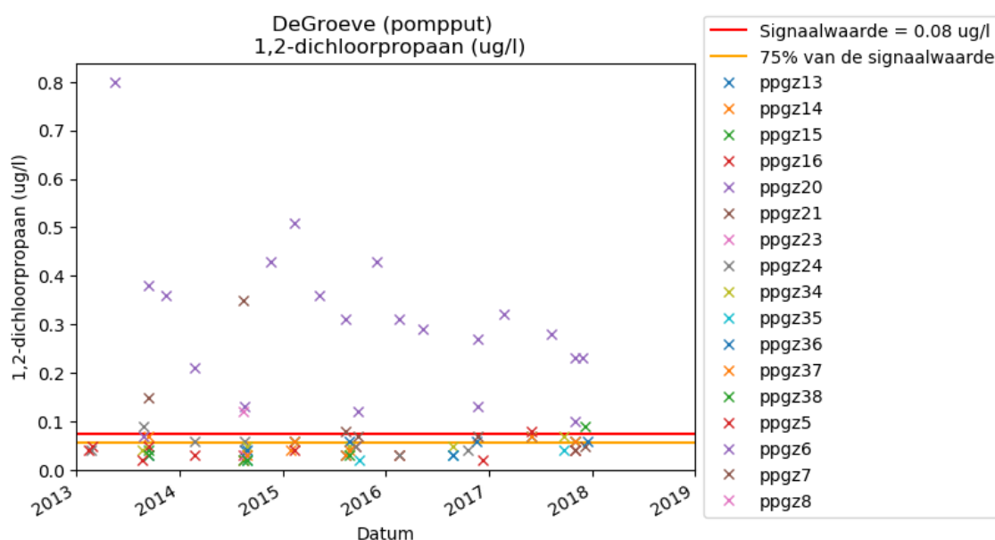
Figuur 5-5 Ontwikkeling 1,2-dichloorpropan pomputten
