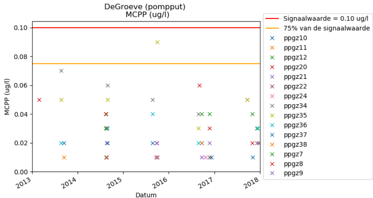
Figuur 5-4 Ontwikkeling MCP pomputten
