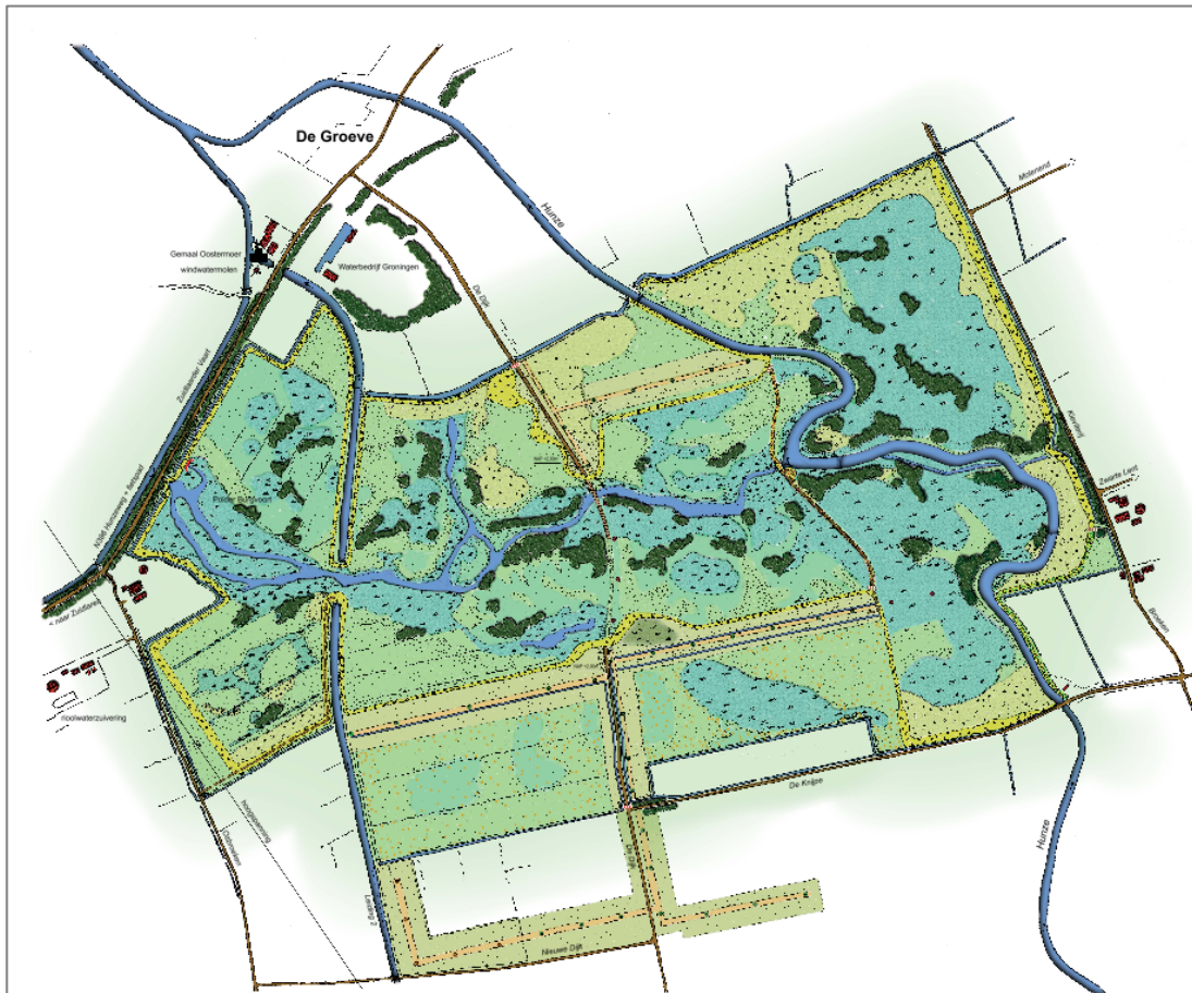
Figuur 6-8 Schetsontwerp Tusschenwater (Waterschap Hunze en Aa's)
