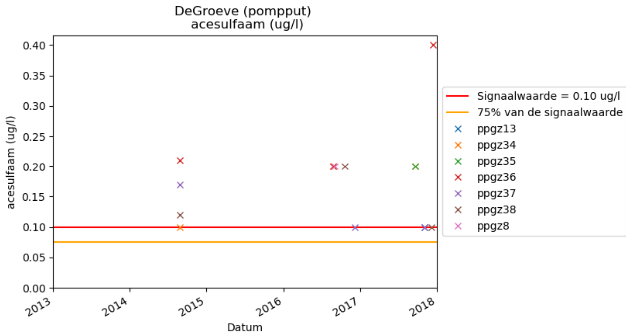
Figuur 5-6 Ontwikkeling acesulfaam pompputten
