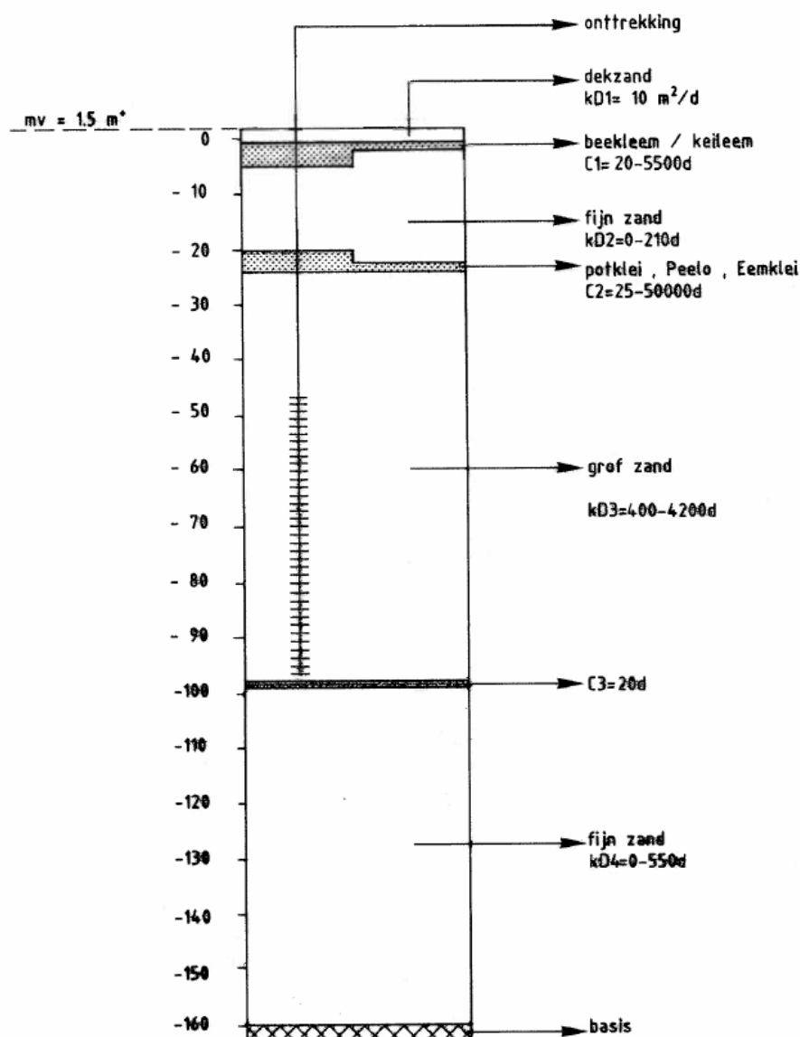
Figuur 4-2 Schematische weergave van de ondergrond ter plaatse van de grondwaterwinning
