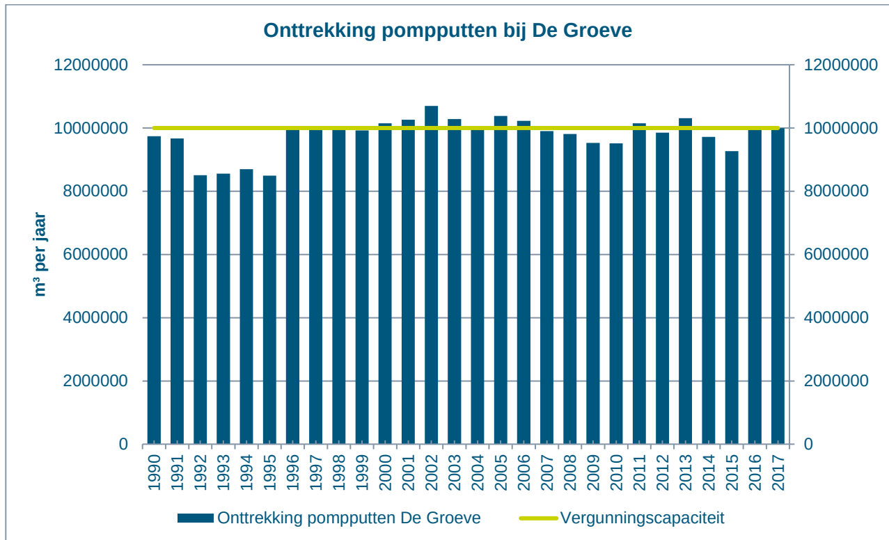
Figuur 2-3 Hoeveelheid werkelijk onttrokken grondwater bij De Groeve
