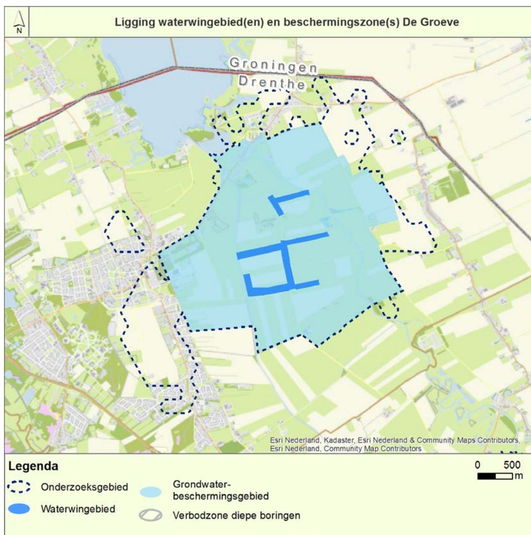
Figuur 2-1 Ligging waterwingebied en grondwaterbeschermingsgebied grondwaterwinning De Groeve
