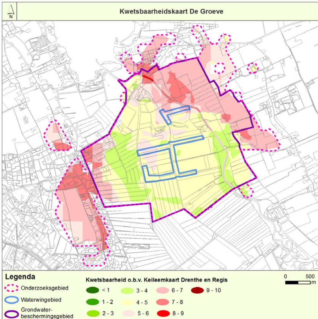
Figuur 4-5 Kwetsbaarheid bovengrond, vastgesteld met de REFLECT-methodiek (2018)
