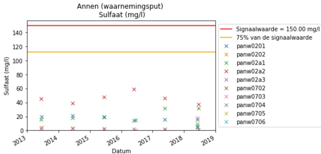
Figuur 5-5 Sulfaatgehalte meetnet
