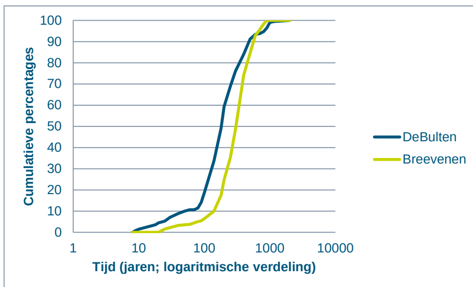
Figuur 4-4 Responsecurves Annen-De Bulten en Annen-Breevenen (Royal Haskoning, 2003)
