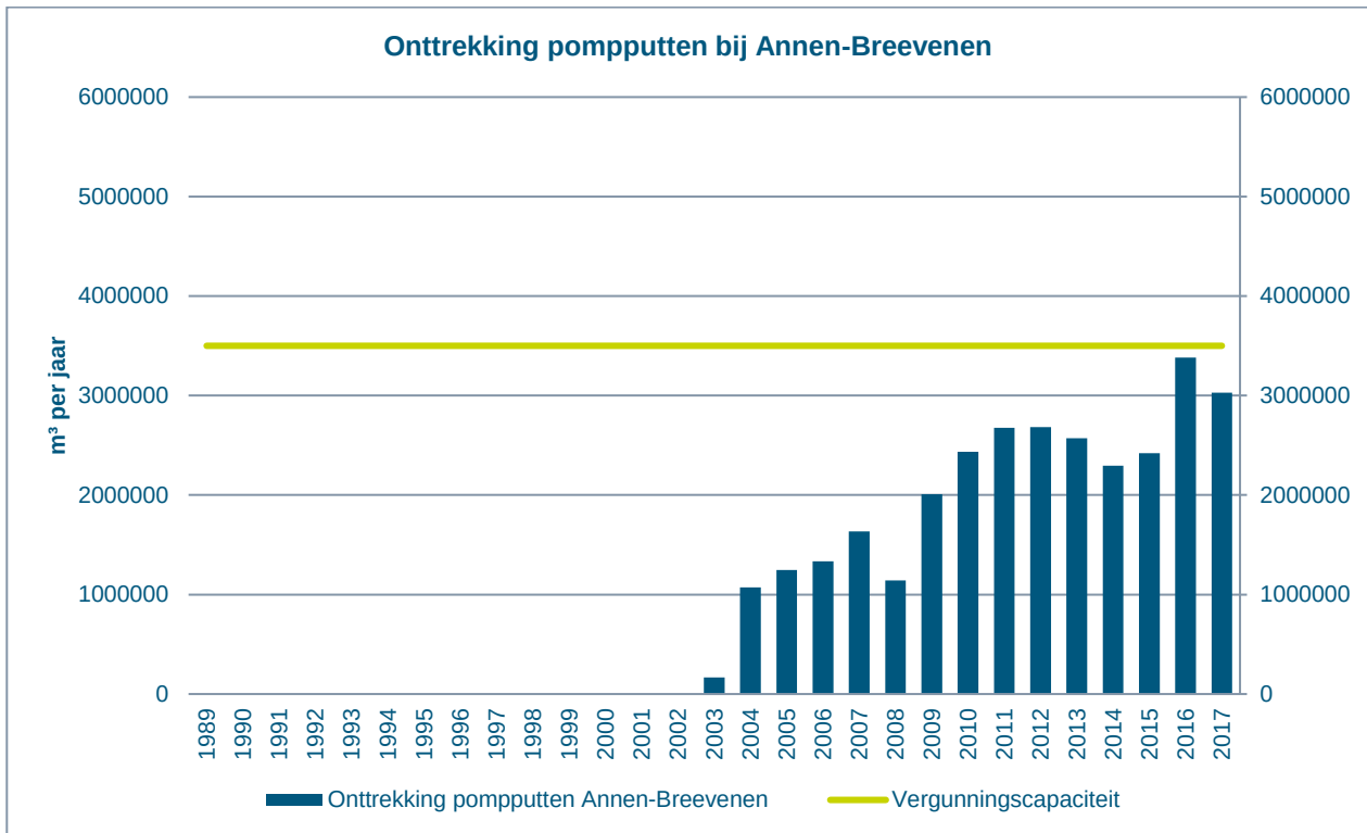
Figuur 2-4 Hoeveelheid werkelijk onttrokken grondwater bij Annen-Breevenen
