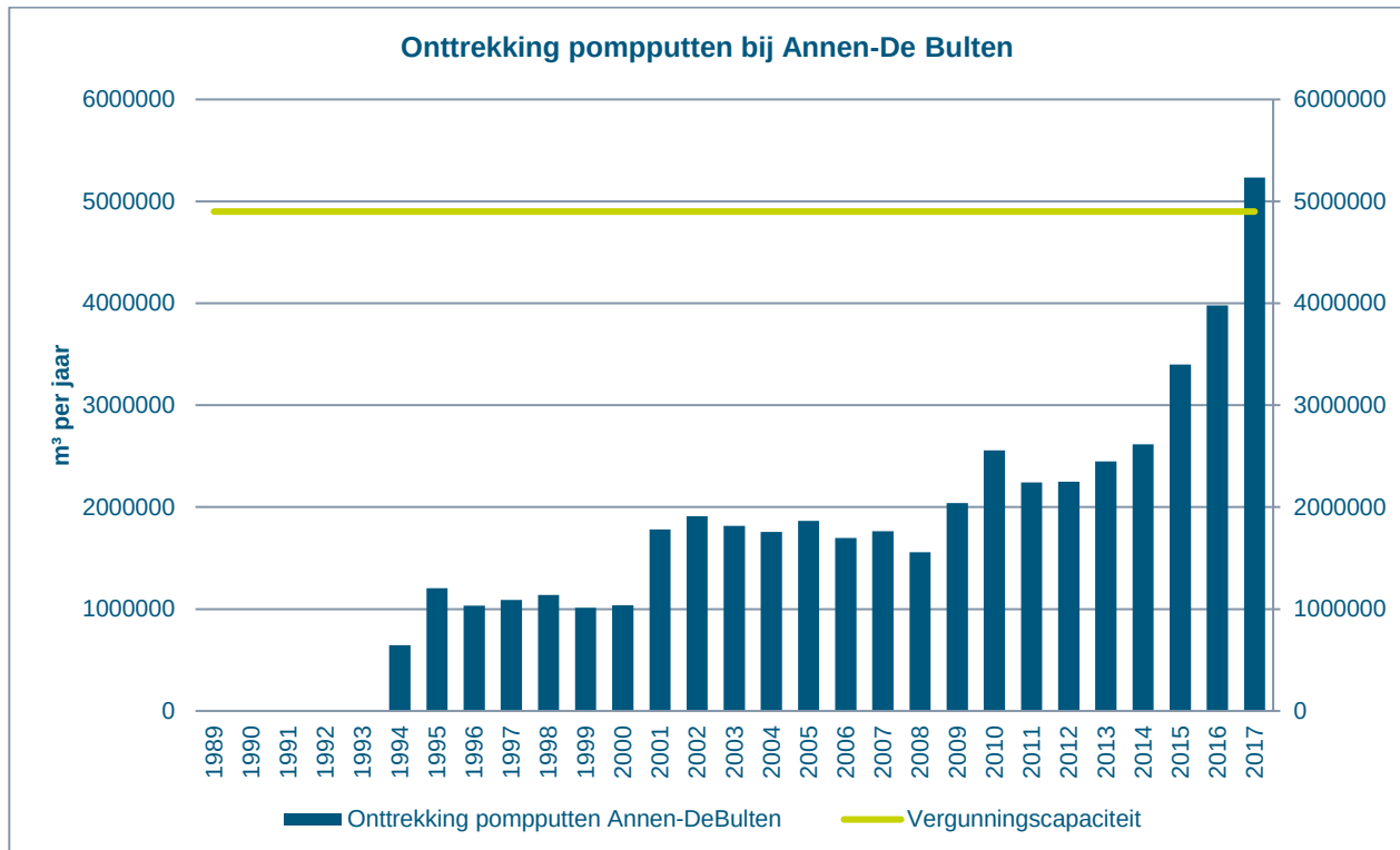
Figuur 2-3 Hoeveelheid werkelijk onttrokken grondwater bij Annen-De Bulten
