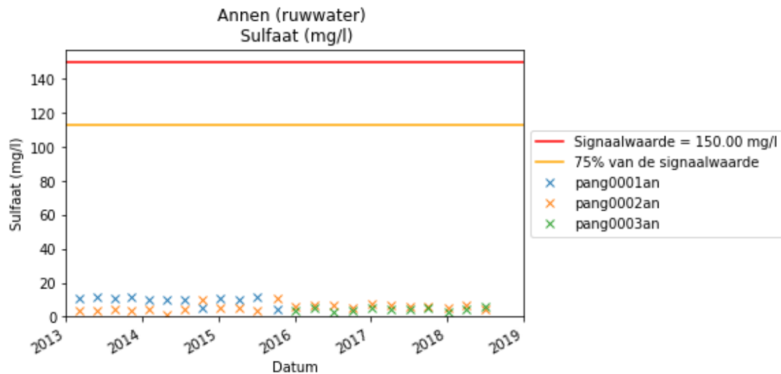
Figuur 5-3 Sulfaatgehalte gezamenlijk ruwwater
