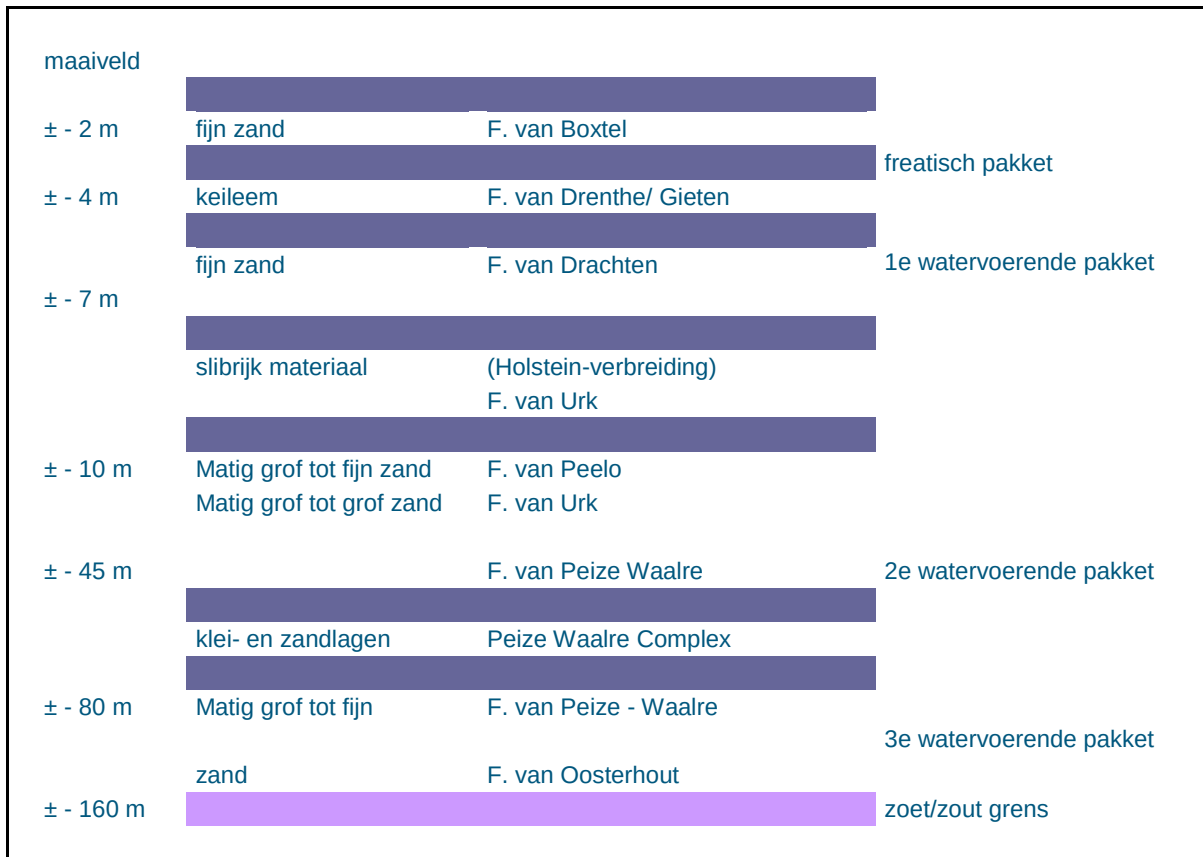
Figuur 4-1 Schematische weergave van de ondergrond ter plaatse van de grondwaterwinning
