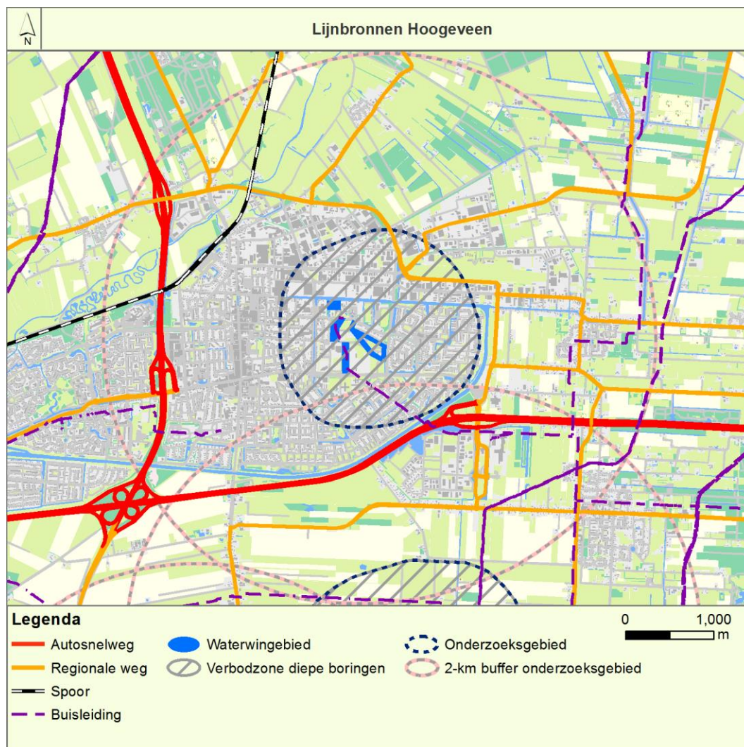
Figuur 6-3 Lijnbronnen
