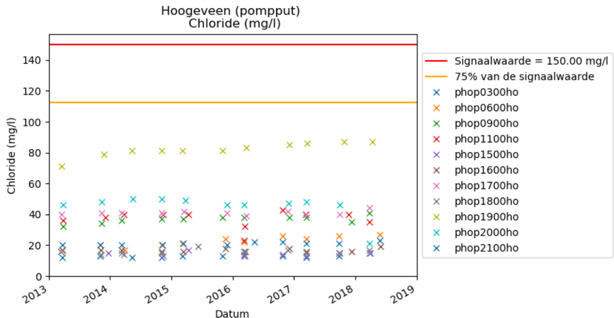
Figuur 5-1 Chloride-gehalte winputten
