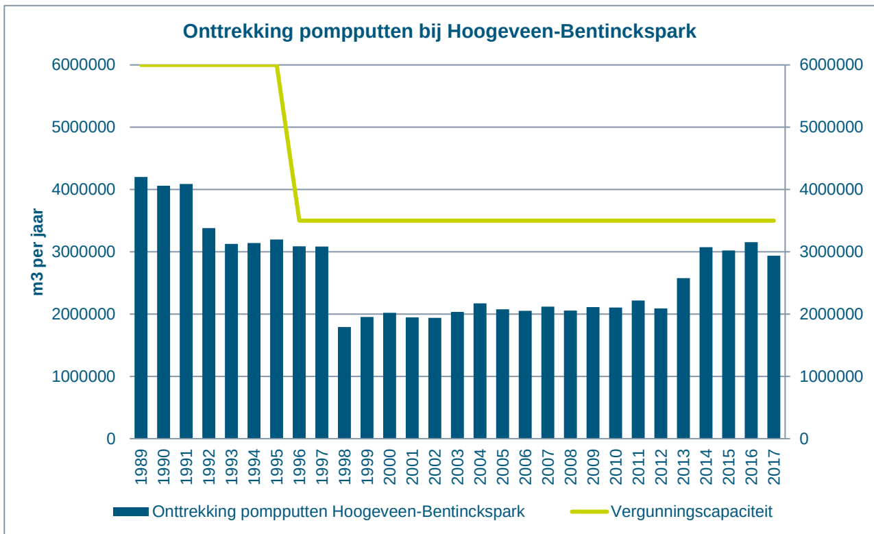
Figuur 2-3 Hoeveelheid werkelijk onttrokken grondwater bij Hoogeveen
