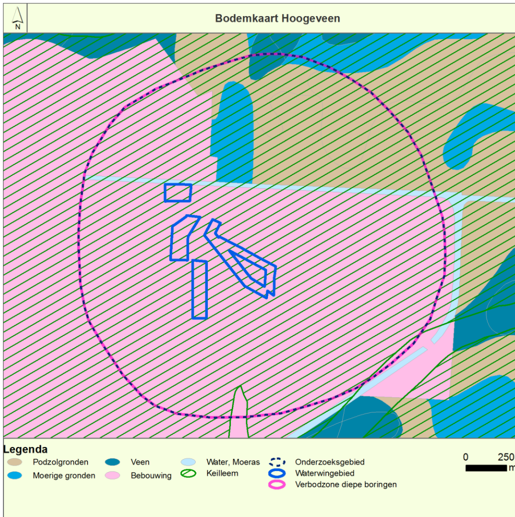
Figuur 4-2 Bodemkaart van het onderzoeksgebied (bron: BasisRegistratieOndergrond (BRO))
