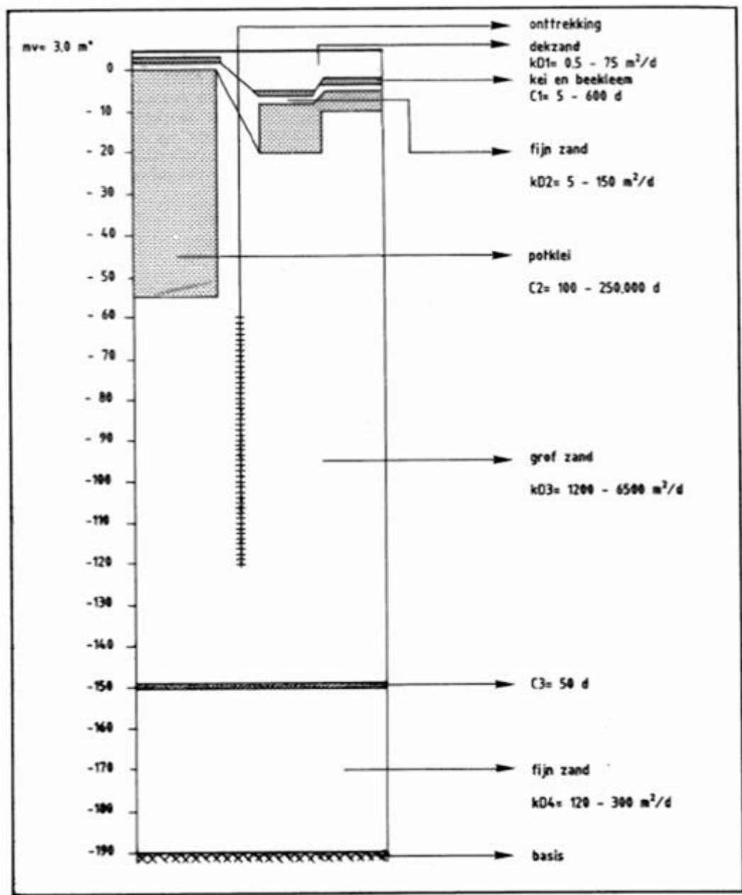
Figuur 4-2 Schematische weergave van de ondergrond ter plaatse van de grondwaterwinning
