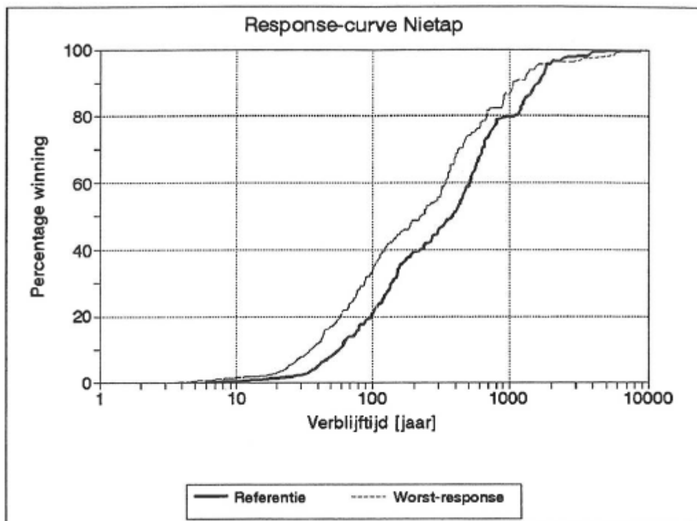
Figuur 4-4 Responsecurve Nietap (IWACO, 1993)
