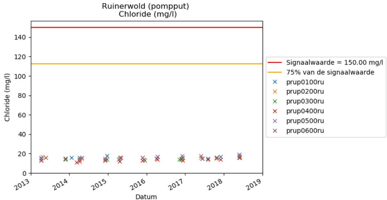
Figuur 5-1 Ontwikkeling chloride
