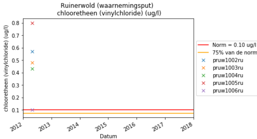
Figuur 5-4 Vinylchloride in het meetnet
