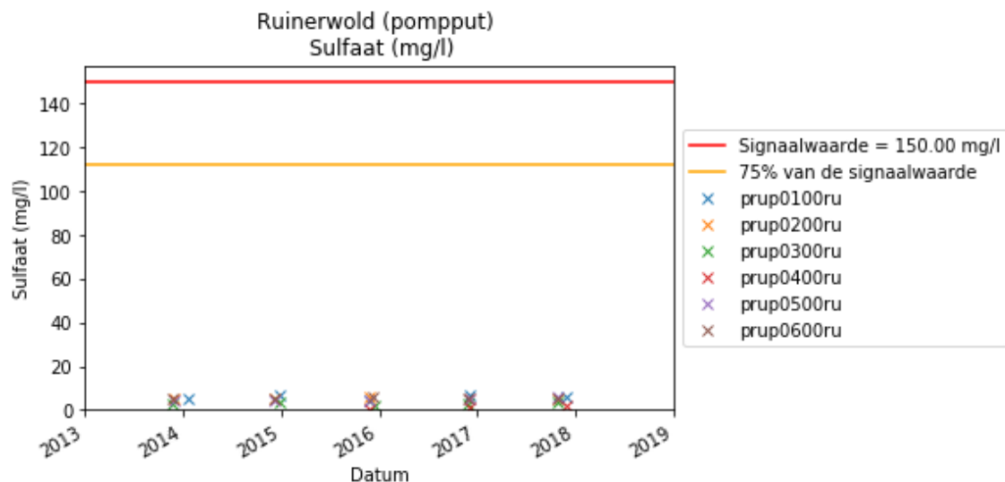
Figuur 5-2 Sulfaatgehalte winputten
