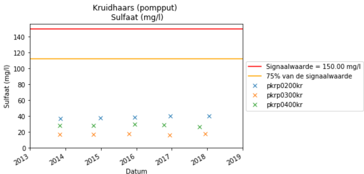
Figuur 5-2 Sulfaatgehalte winputten
