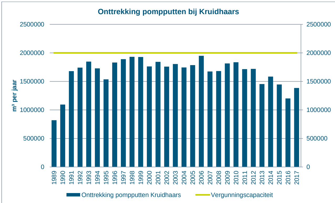
Figuur 2-3 Hoeveelheid werkelijk onttrokken grondwater bij Kruidhaars
