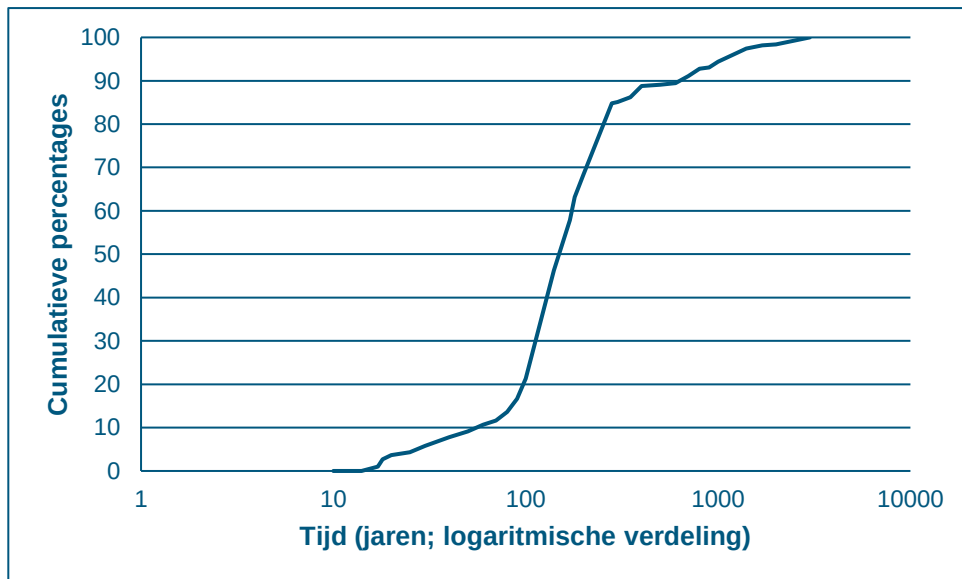
Figuur 4-3 Responsecurve Kruidhaars (IWACO, 1993)
