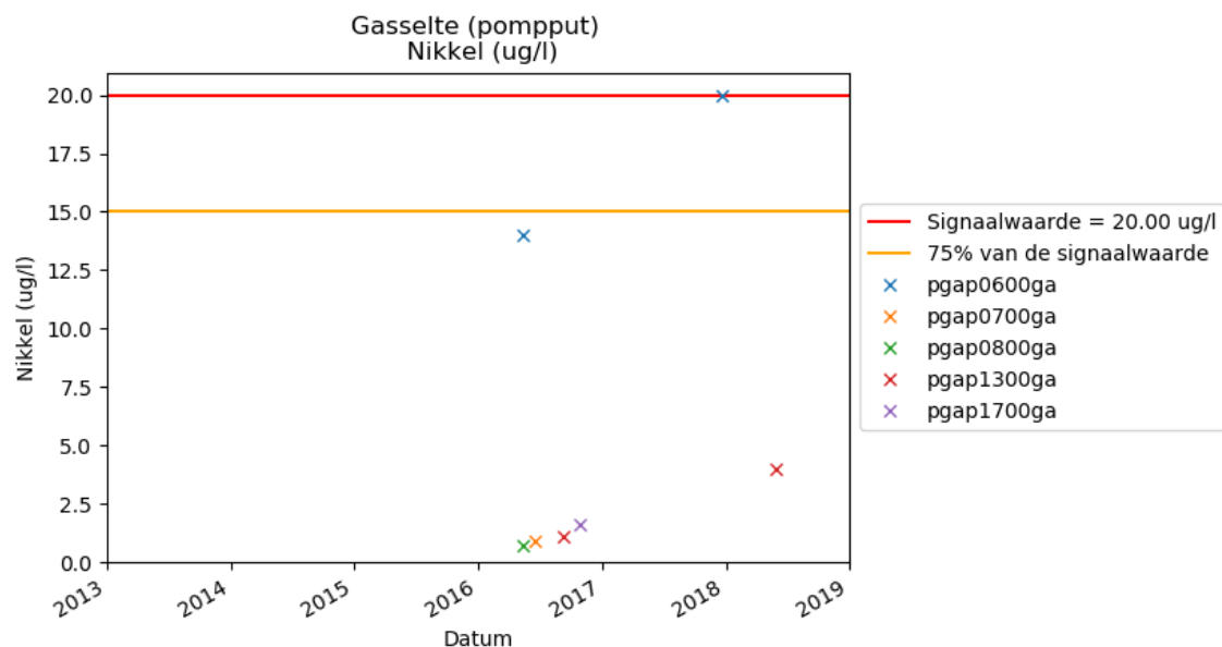
Figuur 5-5 Ontwikkeling nikkel pompputten
