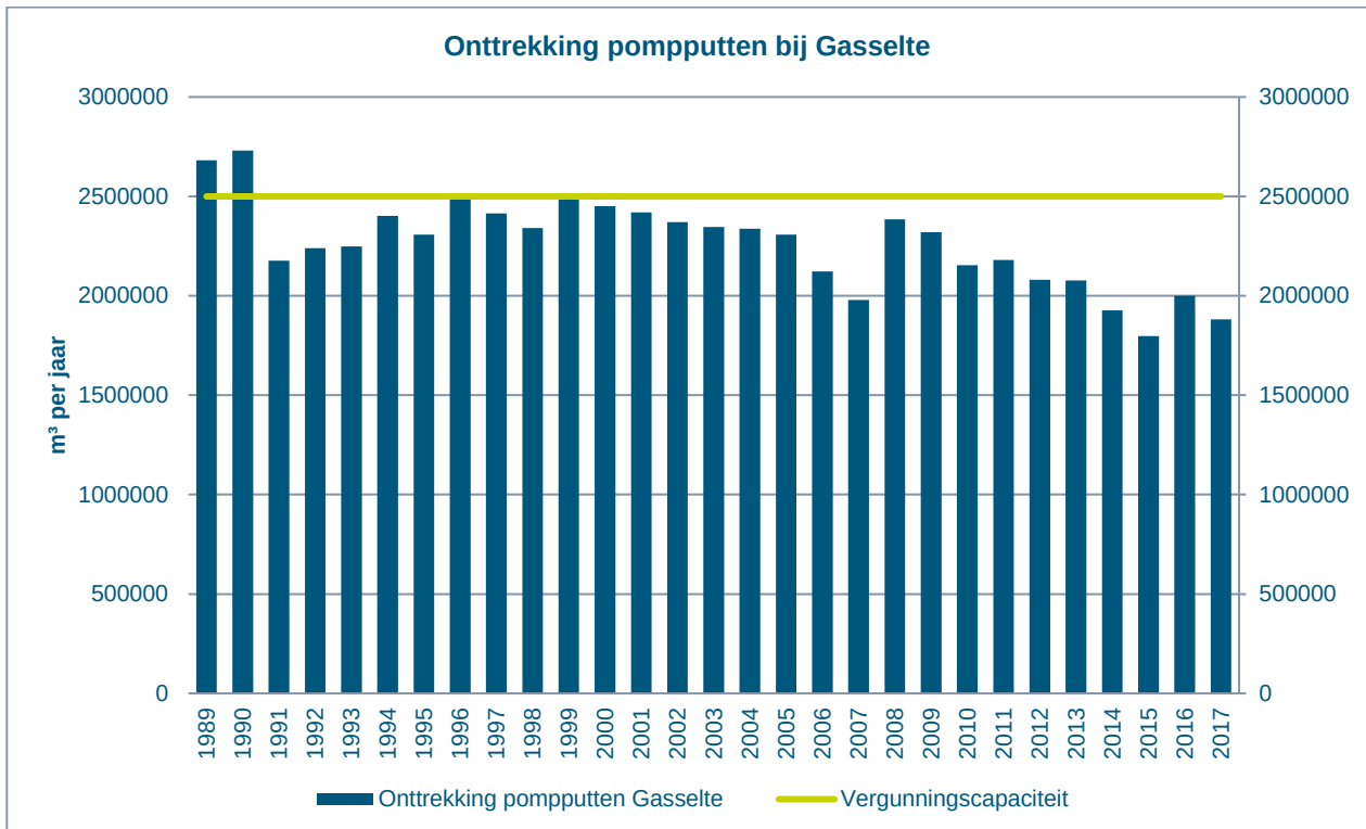
Figuur 2-3 Hoeveelheid werkelijk onttrokken grondwater bij Gasselte
