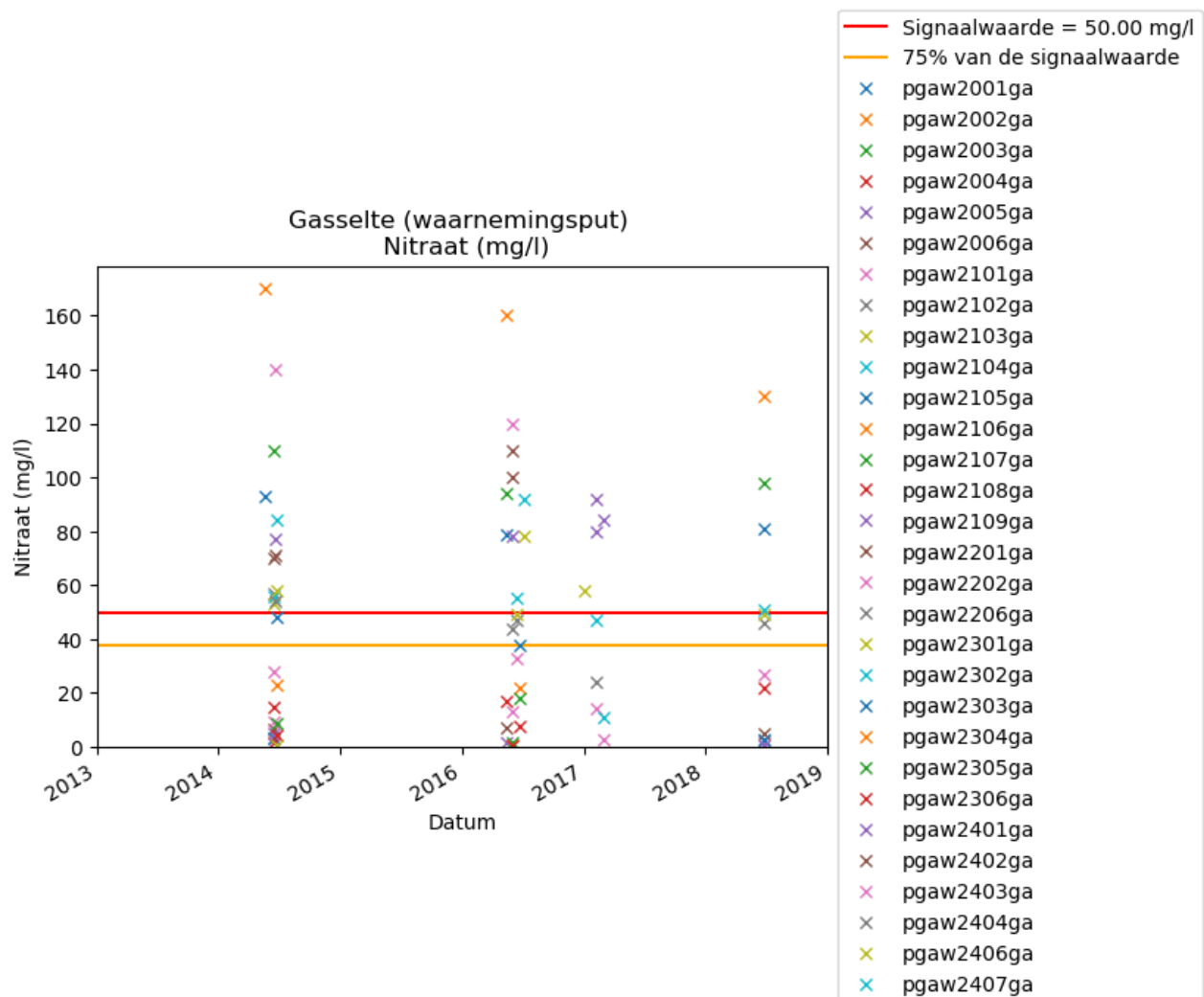
Figuur 5-8 Ontwikkeling nitraat
