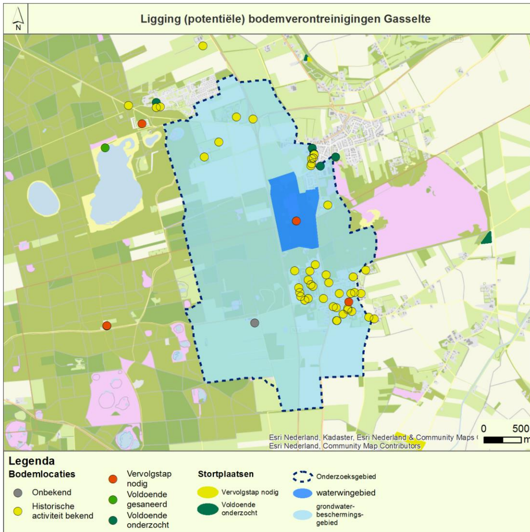
Figuur 6-6 Bodemverontreinigingen
