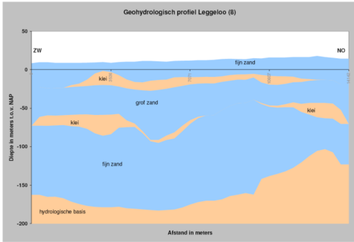
Figuur 4-2 Schematische weergave van de ondergrond ter plaatse van de grondwaterwinning
