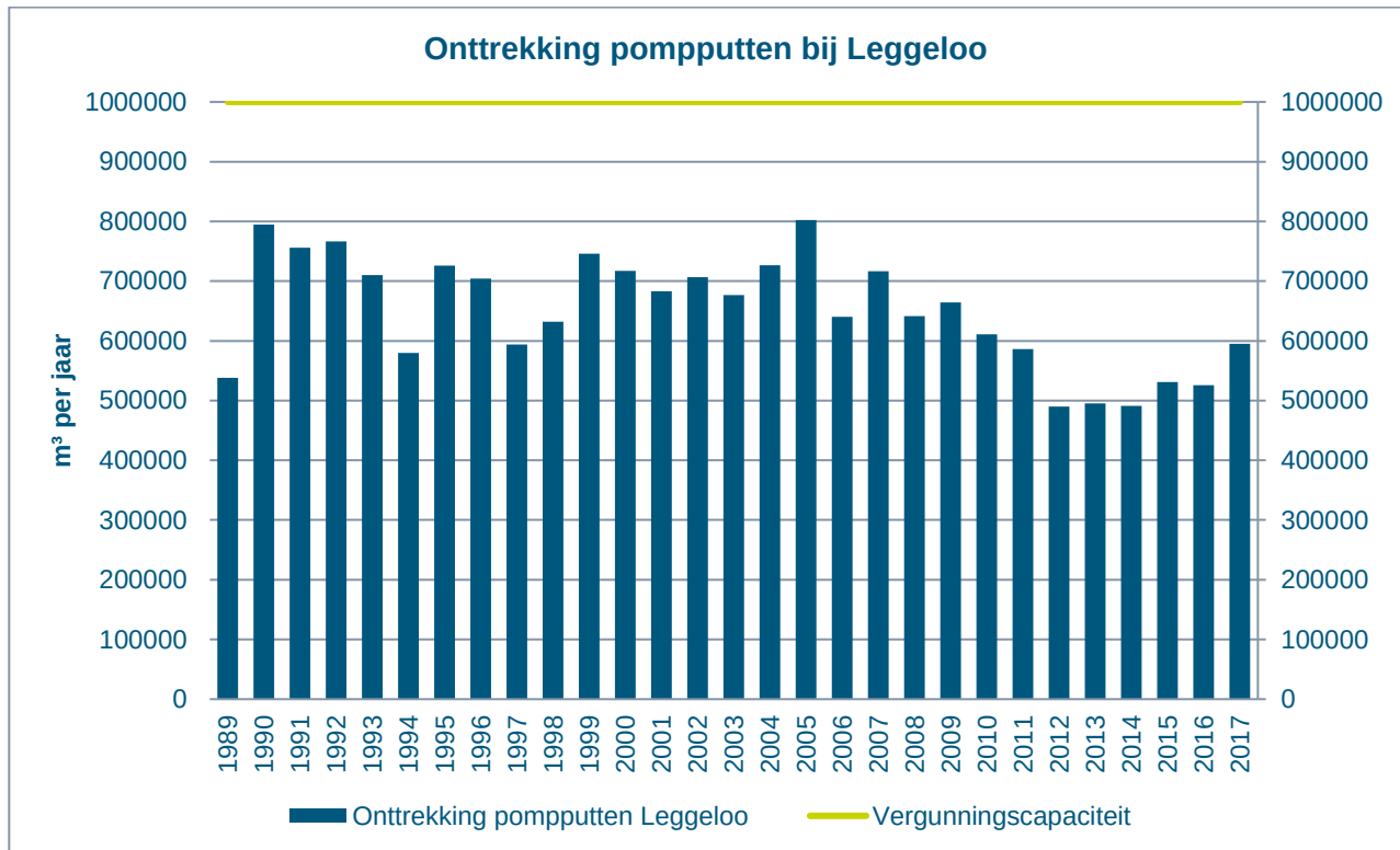
Figuur 2-3 Hoeveelheid werkelijk onttrokken grondwater bij Leggeloo
