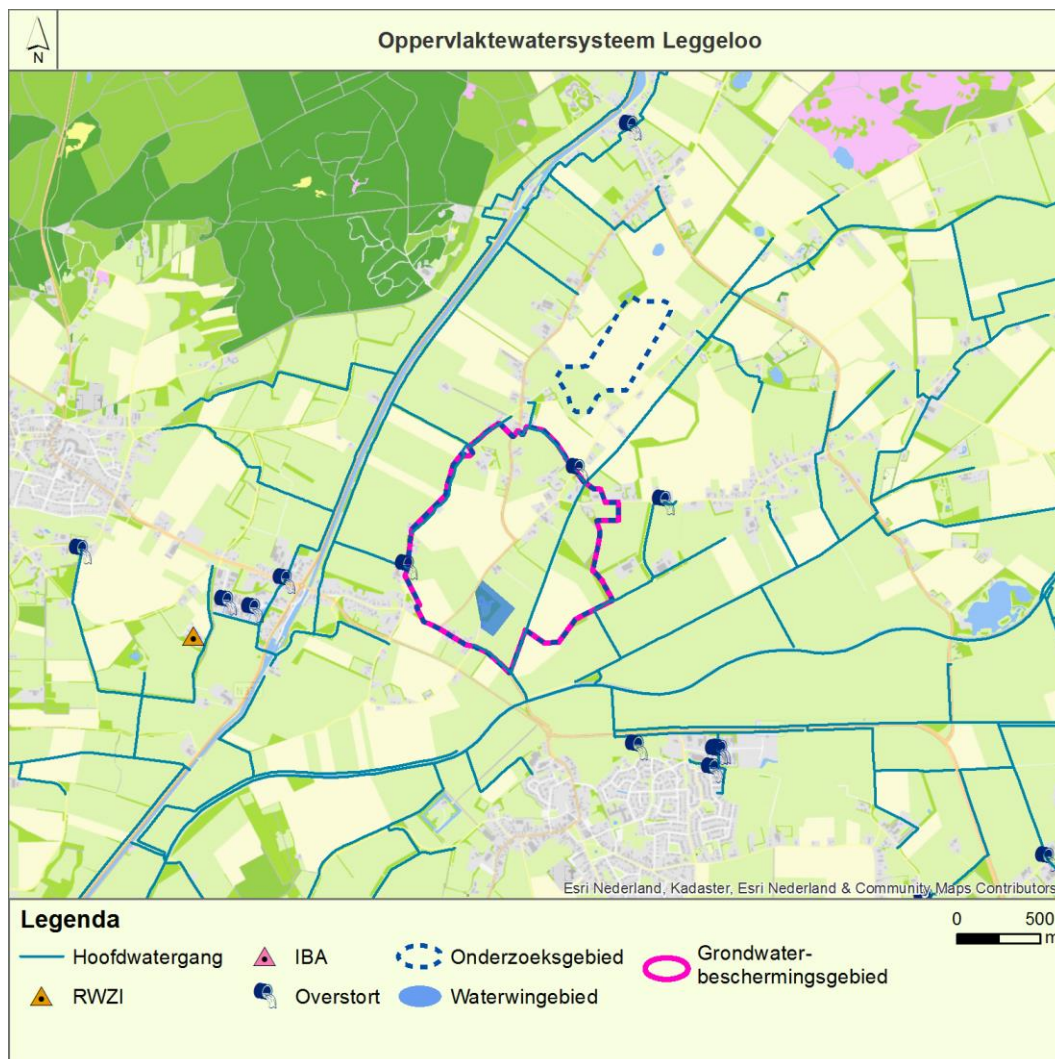
Figuur 6-4 Oppervlaktewatersysteem Leggeloo
