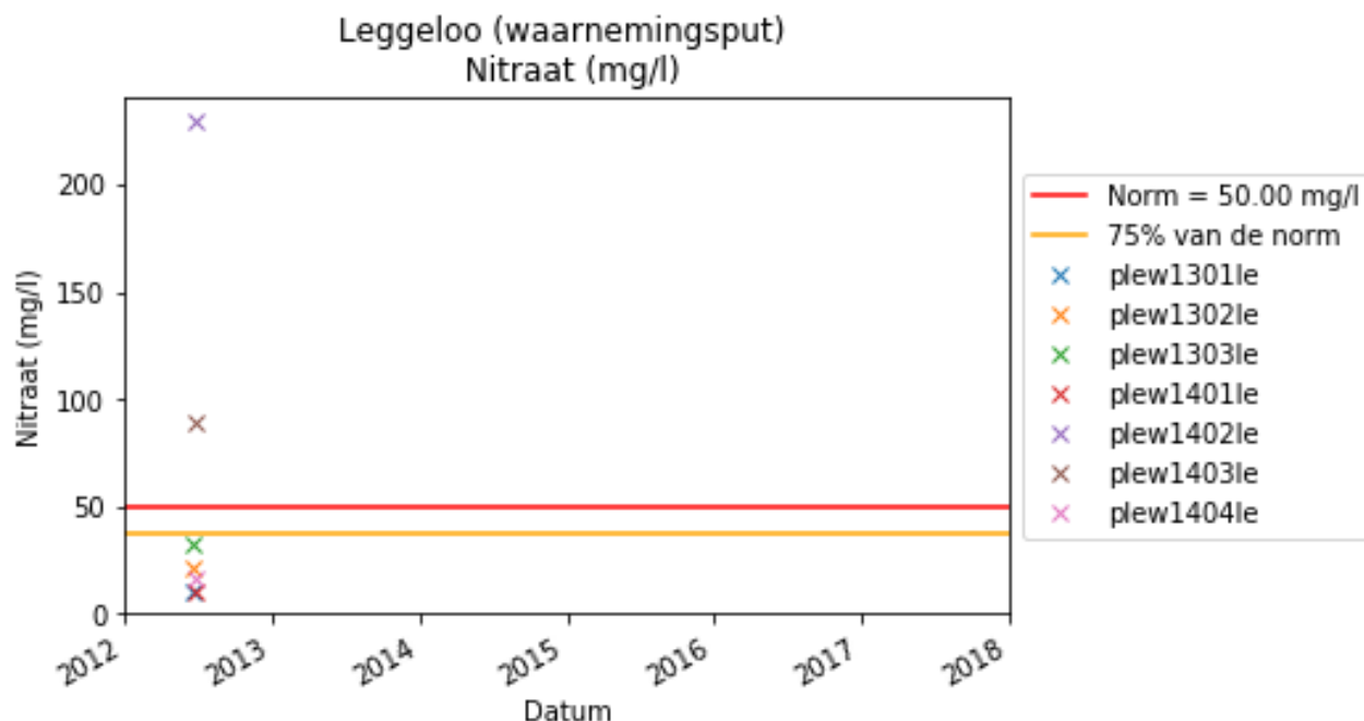
Figuur 5-8 Nitraat concentratie meetnet
