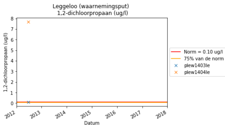
Figuur 5-9 Ontwikkeling 1,2-dichloorpropaan meetnet
