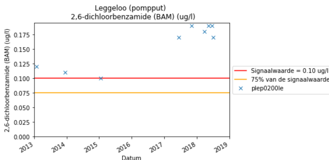
Figuur 5-3 Ontwikkeling BAM winputten
