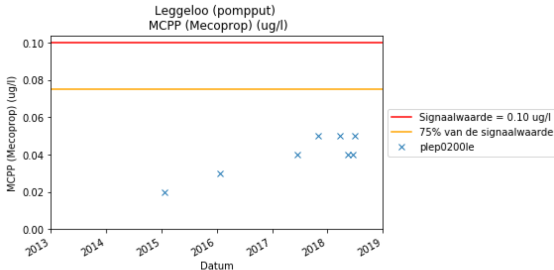
Figuur 5-4 Ontwikkeling MCPP
