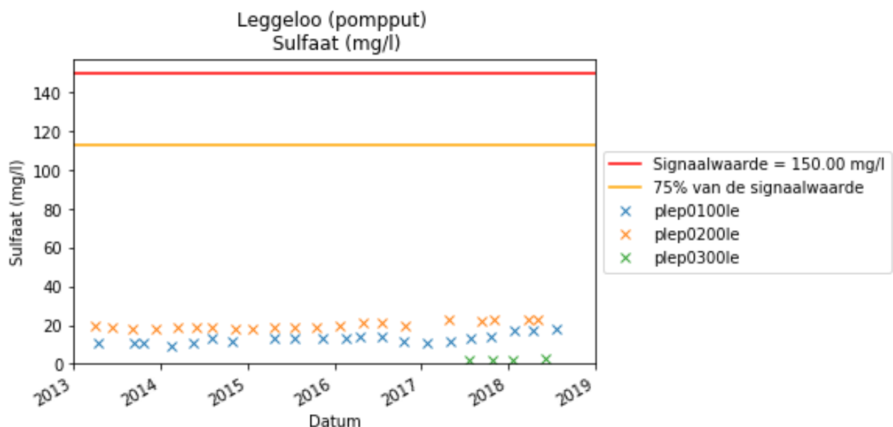
Figuur 5-6 Sulfaatgehalte winputten
