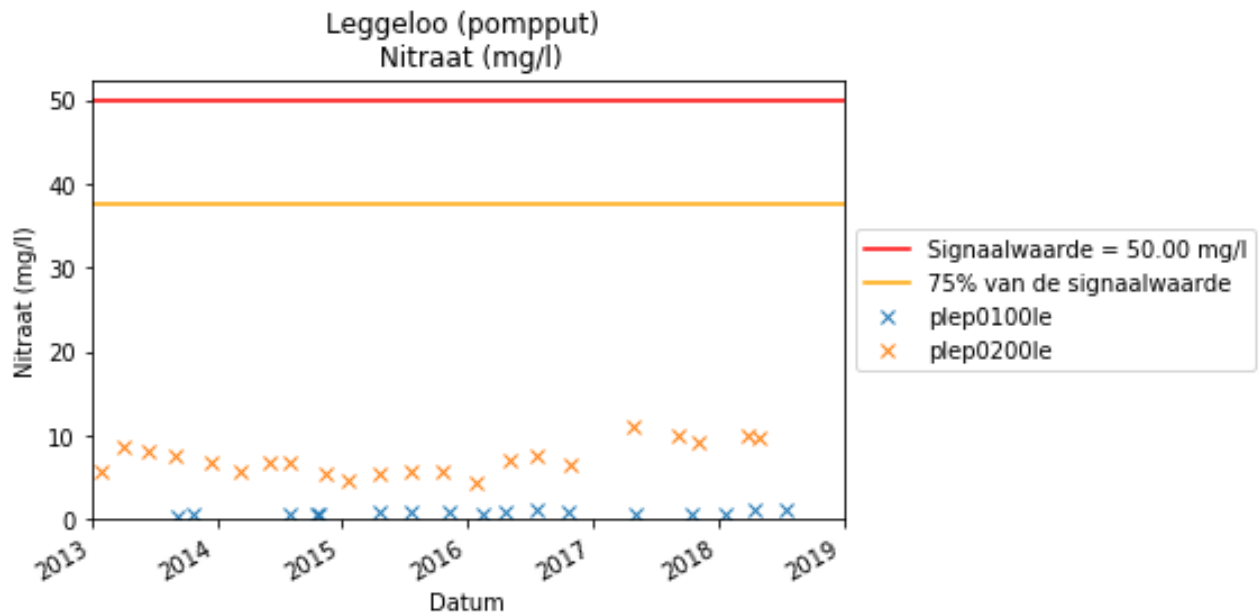
Figuur 5-1 Ontwikkeling nitraat
