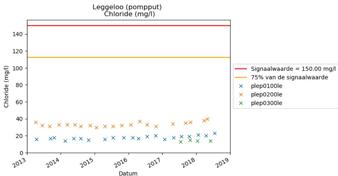
Figuur 5-2 Ontwikkeling chloride
