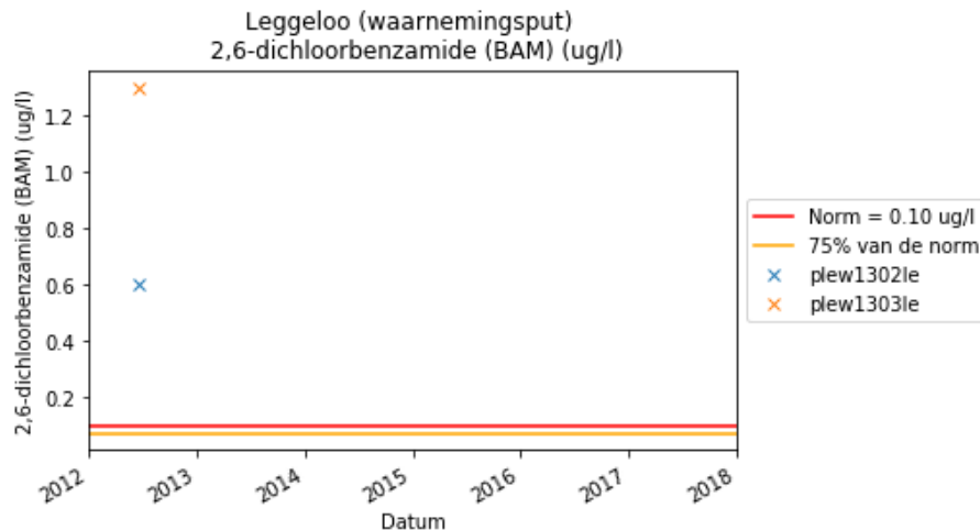
Figuur 5-10 Ontwikkeling BAM meetnet
