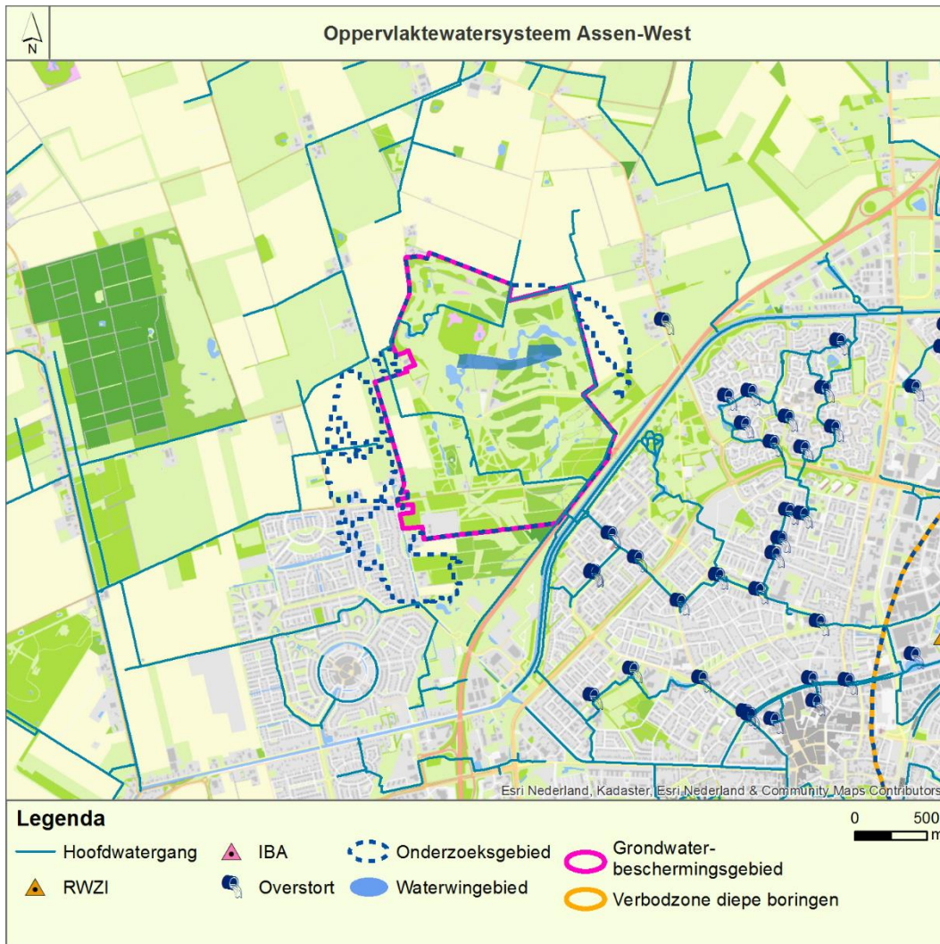
Figuur 6-4 Oppervlaktewatersysteem Assen-West.
