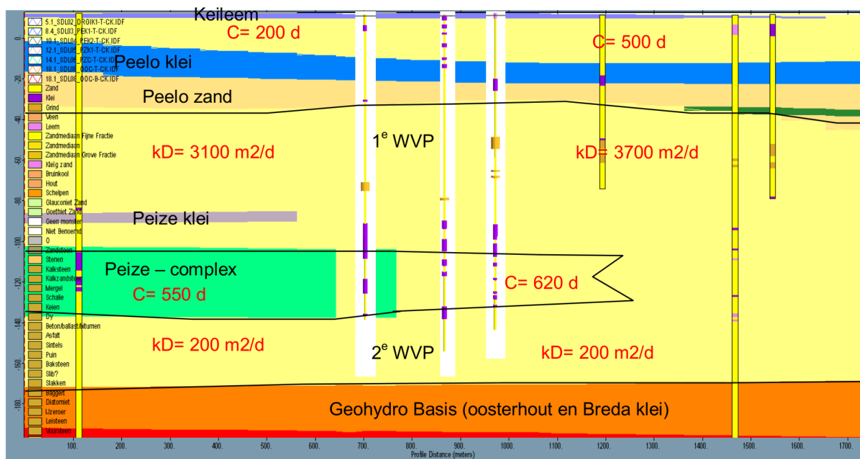
Figuur 4-2 Schematische weergave van de ondergrond ter plaatse van de grondwaterwinning in de noord-zuidrichting (bron Grontmij, 2015).
