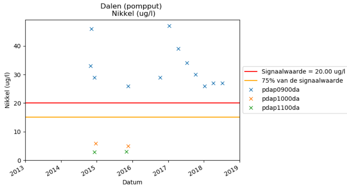
Figuur 5-4 Nikkelgehalte winputten
