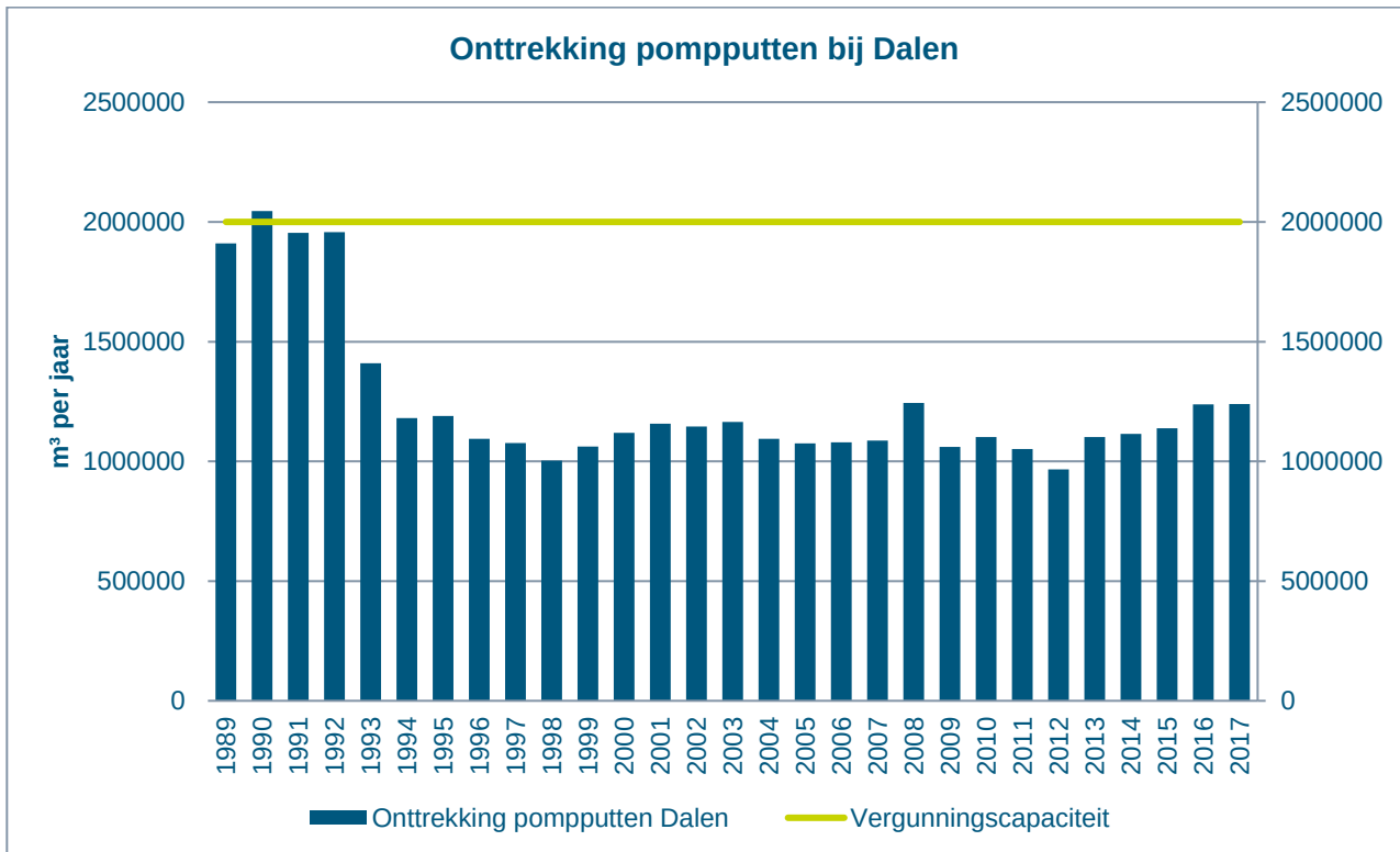
Figuur 2-3 Hoeveelheid werkelijk onttrokken grondwater bij Dalen
