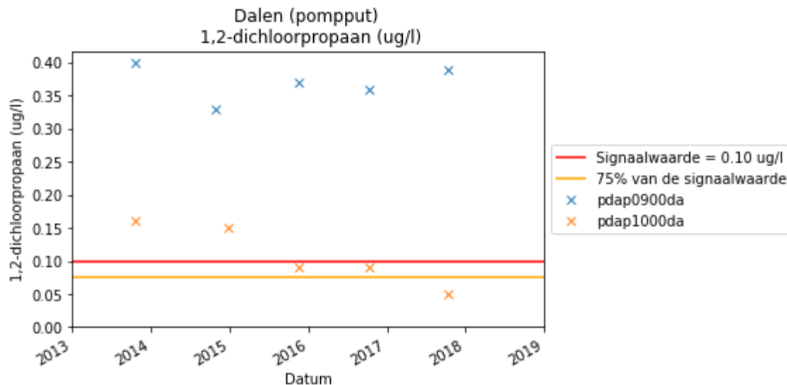
Figuur 5-2 Het concentratie verloop van 1,2-dichloorpropaan over de periode 2012-2018
