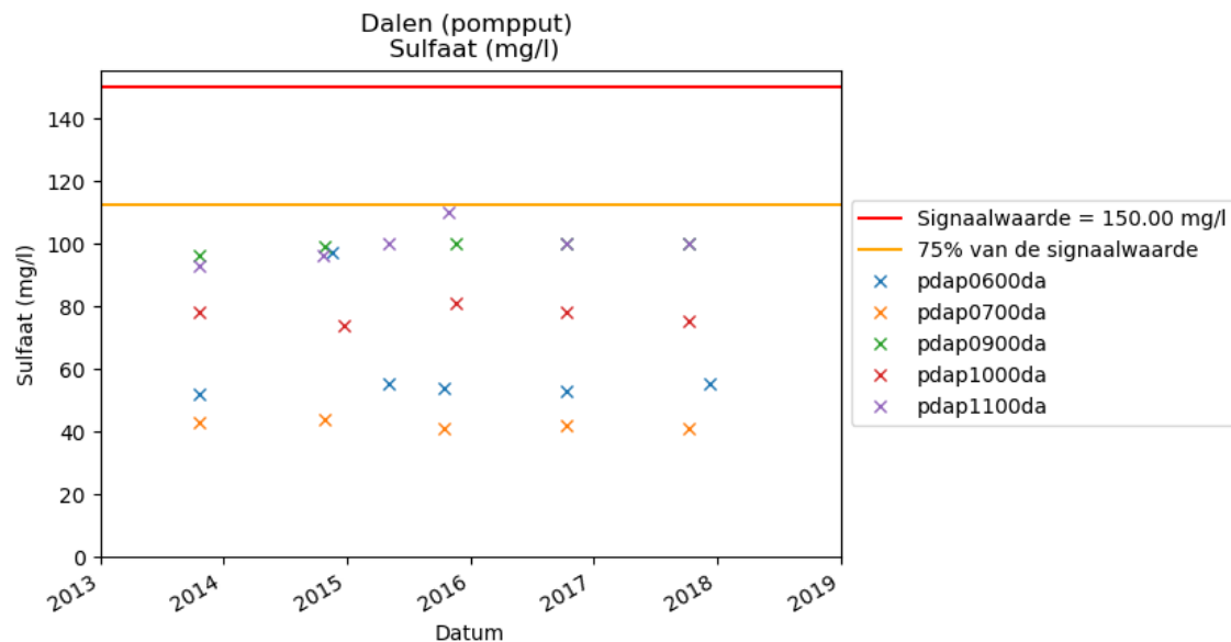
Figuur 5-3 Sulfaatgehalte winputten
