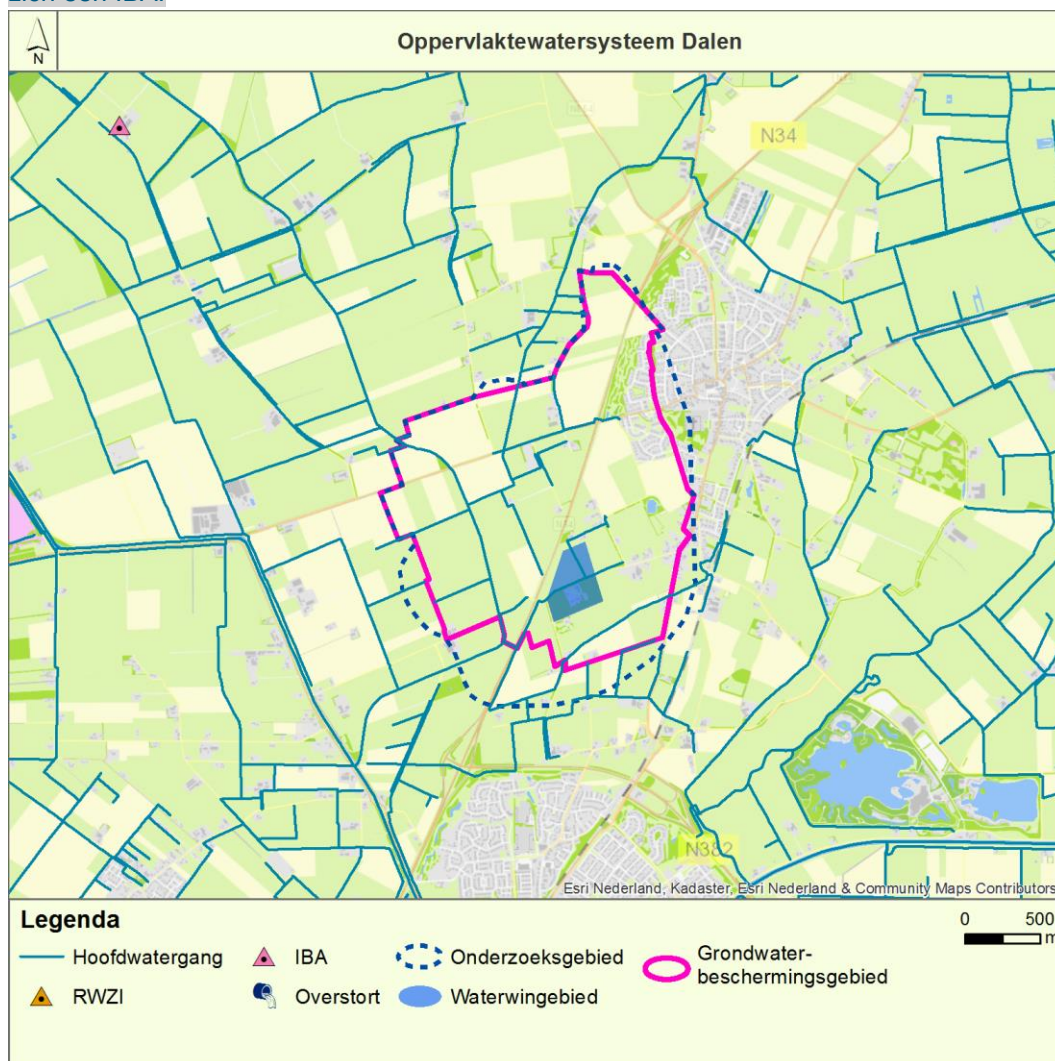
Figuur 6-4 Oppervlaktewatersysteem Dalen
