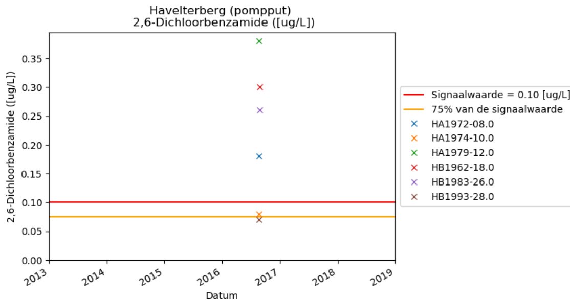
Figuur 5-2 Ontwikkeling BAM winputten
