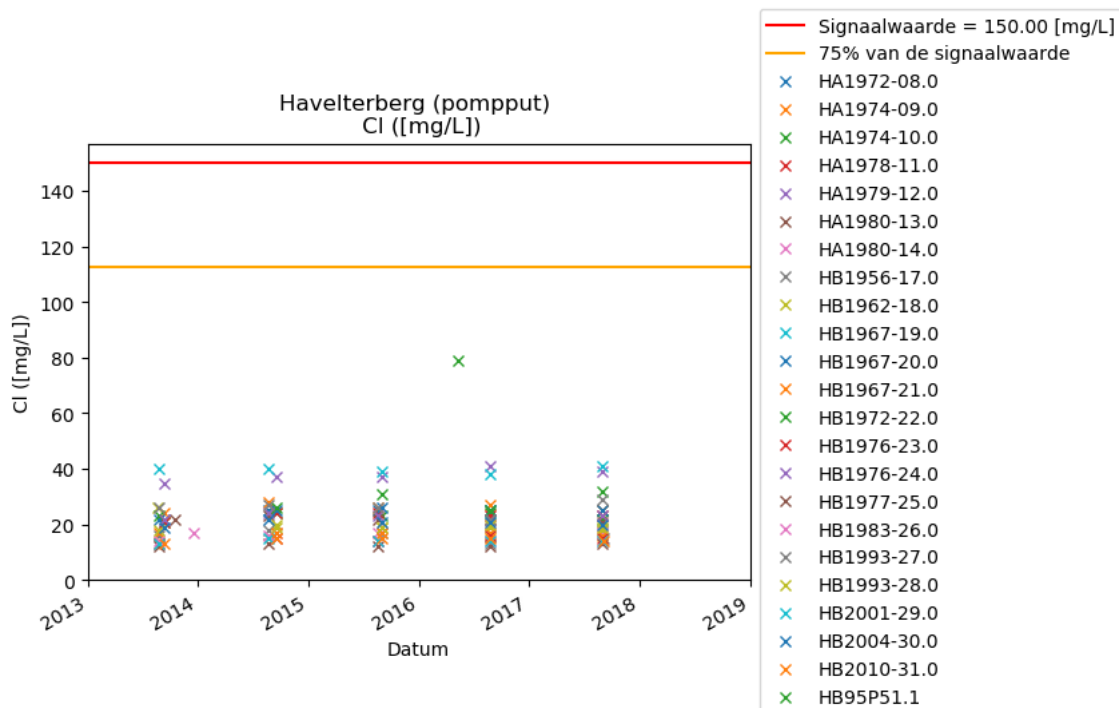
Figuur 5-1 Ontwikkeling chloride
