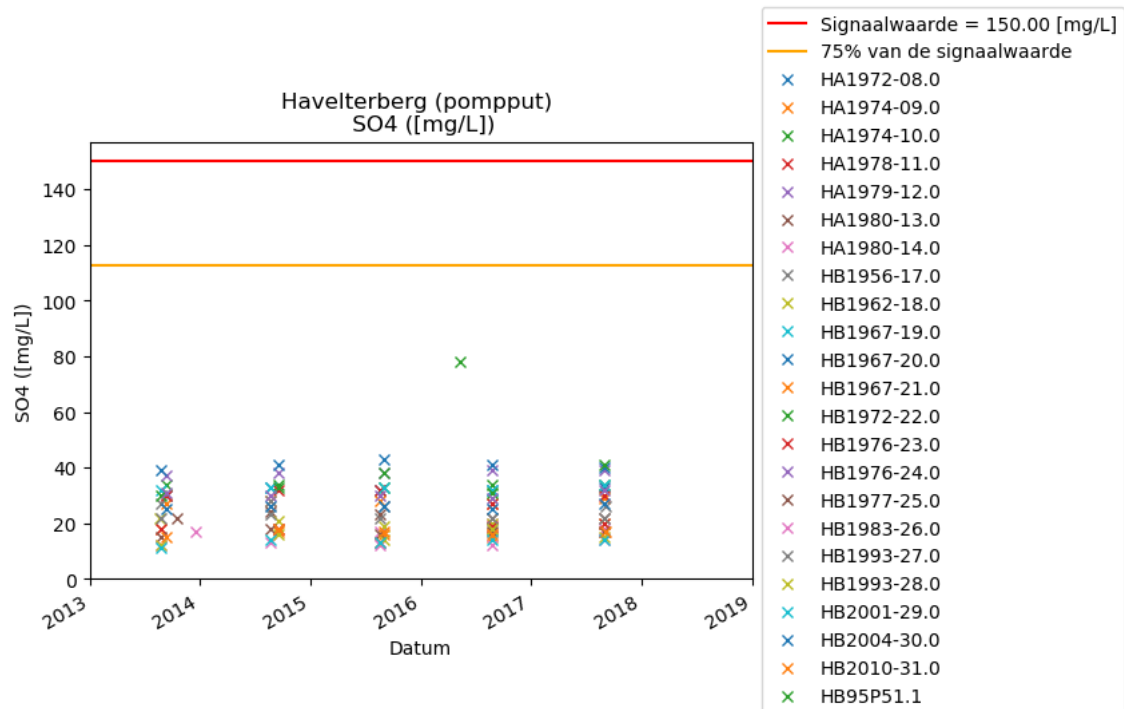
Figuur 5-3 Sulfaatgehalte winputten
