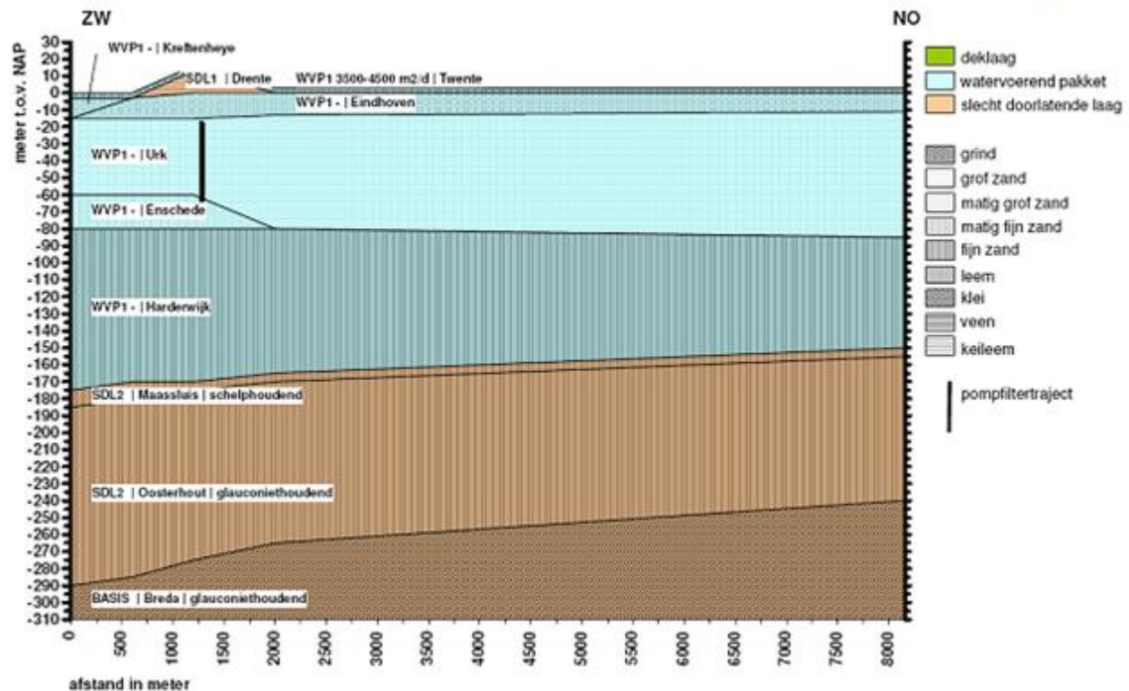
Figuur 4-2 Schematische weergave van de ondergrond ter plaatse van de grondwaterwinning
