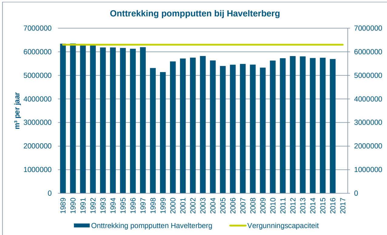
Figuur 2-3 Hoeveelheid werkelijk onttrokken grondwater bij Havelterberg
