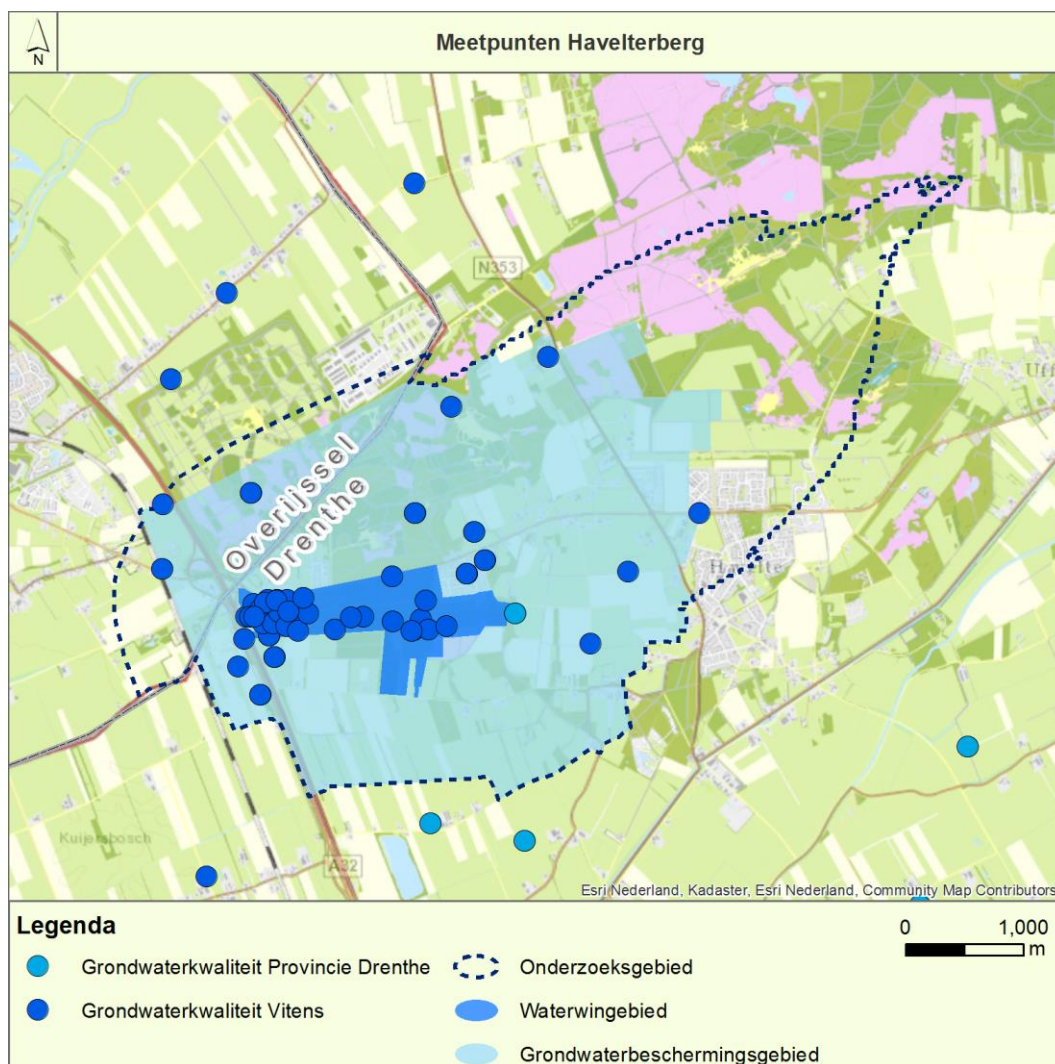
Figuur 5-5 Meetpunten Havelterberg
