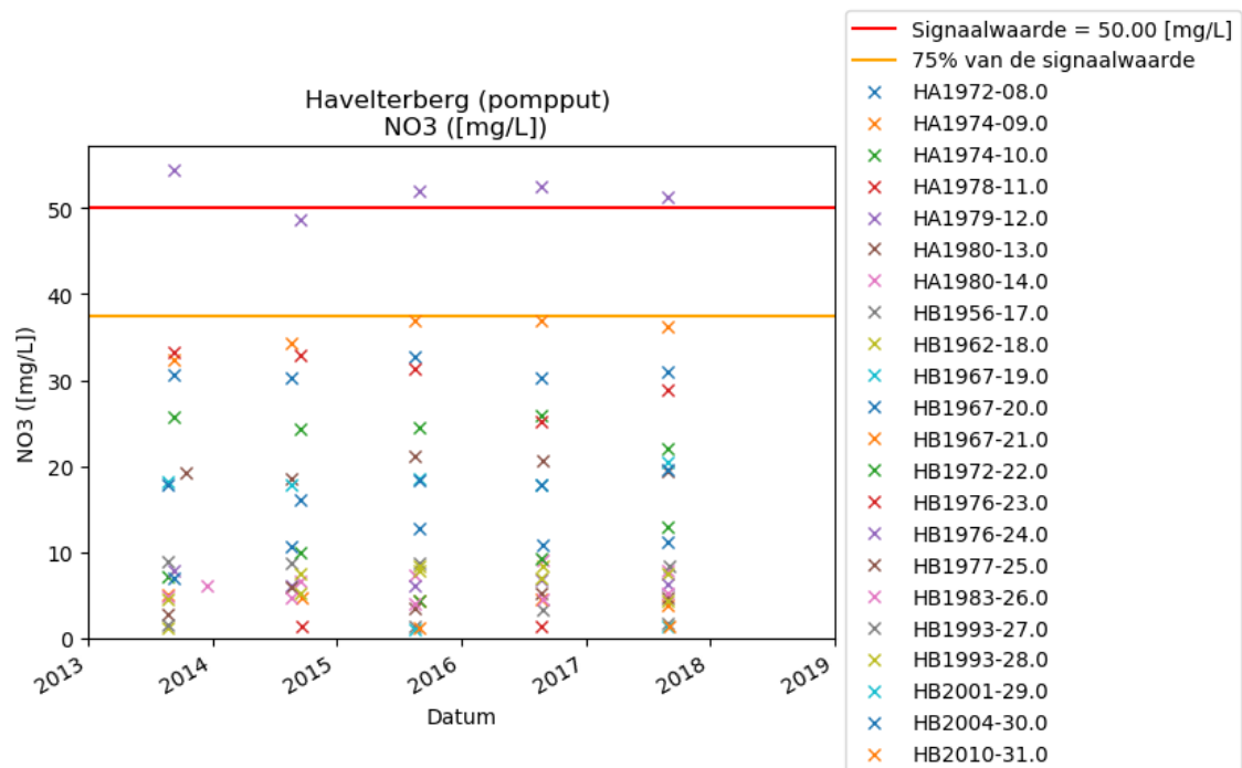
Figuur 5-4 Nitraatgehalte winputten
