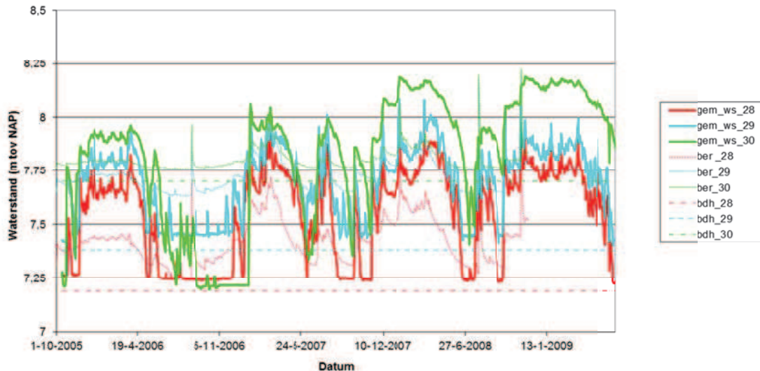
Figuur 30. Waterstanden bij meetpunten ws_28, ws_29 en ws_30
