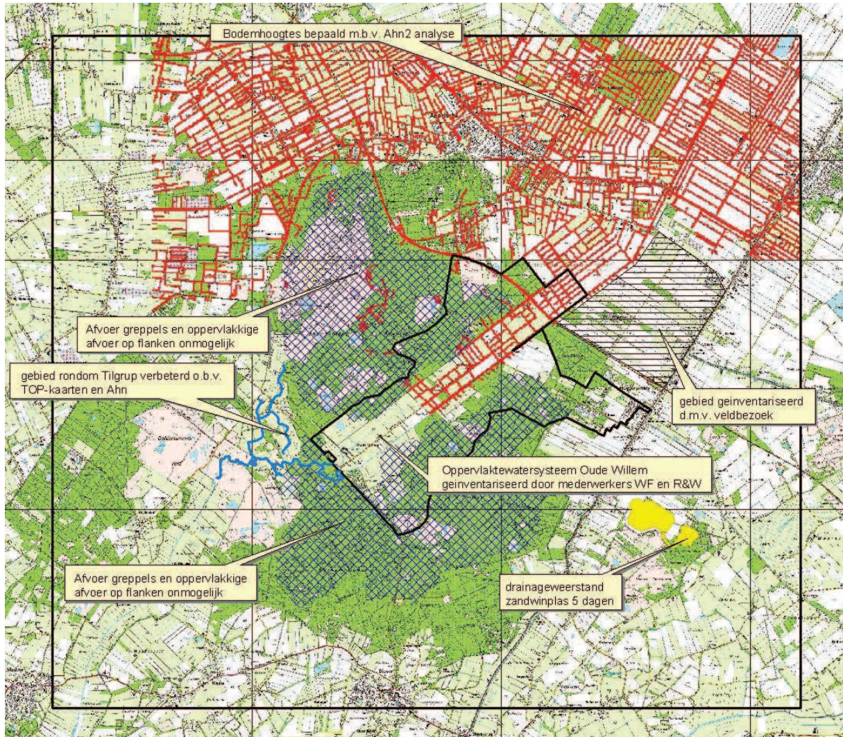
Figuur 6. Overzichtsk kaart wijzigingen aan oppervlaktewatersysteem binnen modelgebied
