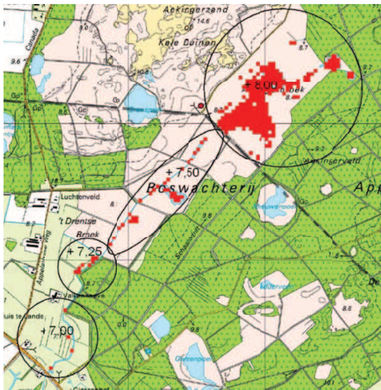
Figuur 24. De stagnatie gebieden in de Vledder Aa en de bijbehorende drempelwaardes
