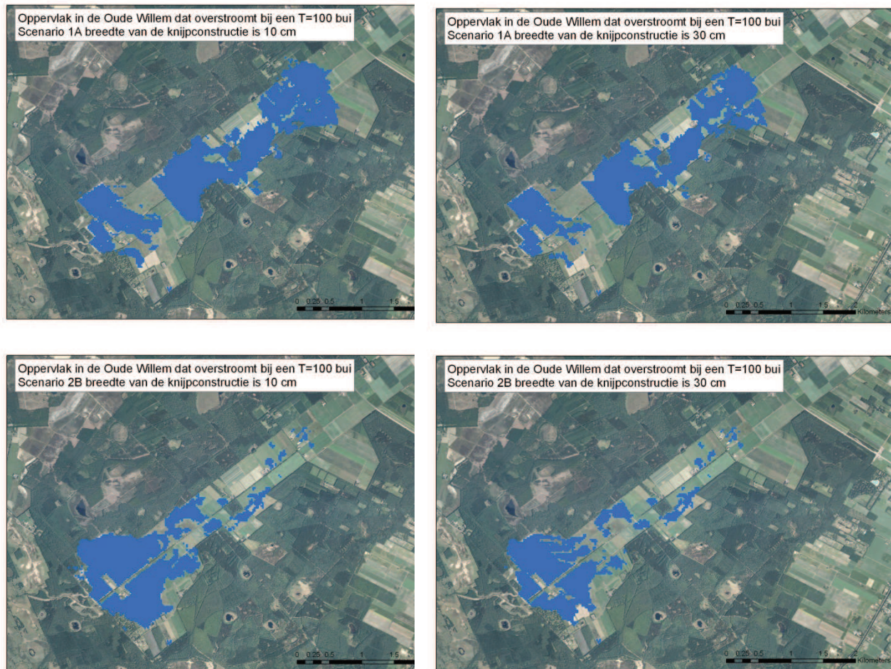
Figuur 40. Oppervlak in de Oude Willem dat overstroomt bij T=100 bui voor scenario 1A en 2B, met resp. 4 en 1 knijpconstructie met een opening van 10 en 30cm
