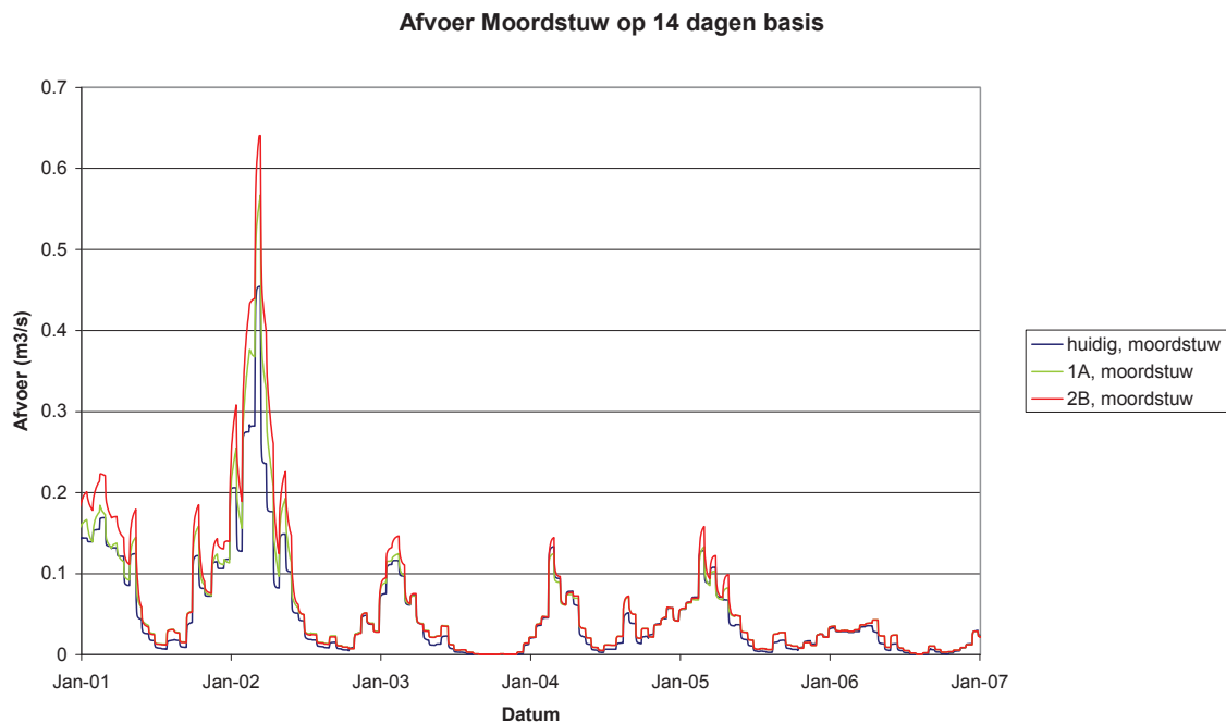
Figuur 43. Afvoer van de Moordstuw in huidige situatie, variant 1A en variant 2B
