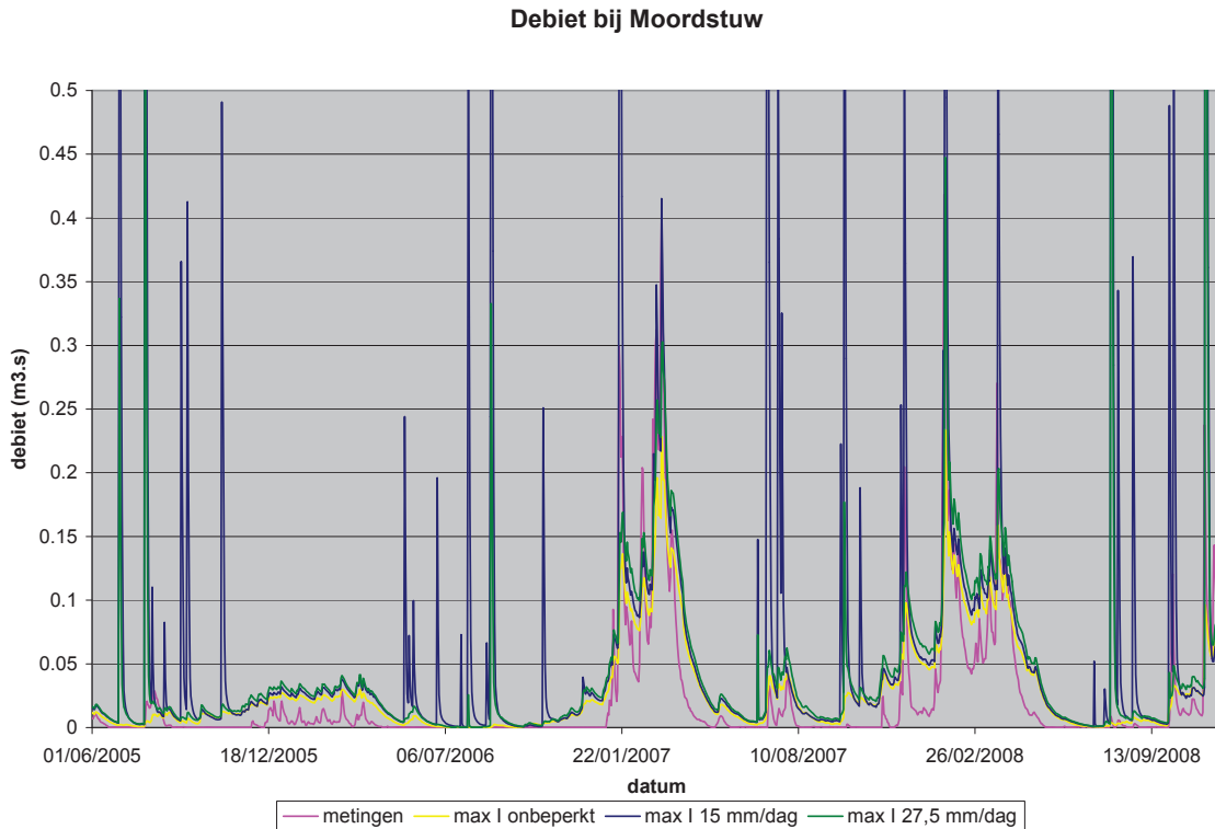
Figuur 27. Afvoer bij de Moordstuw periode augustus 2004 tot december 2009
