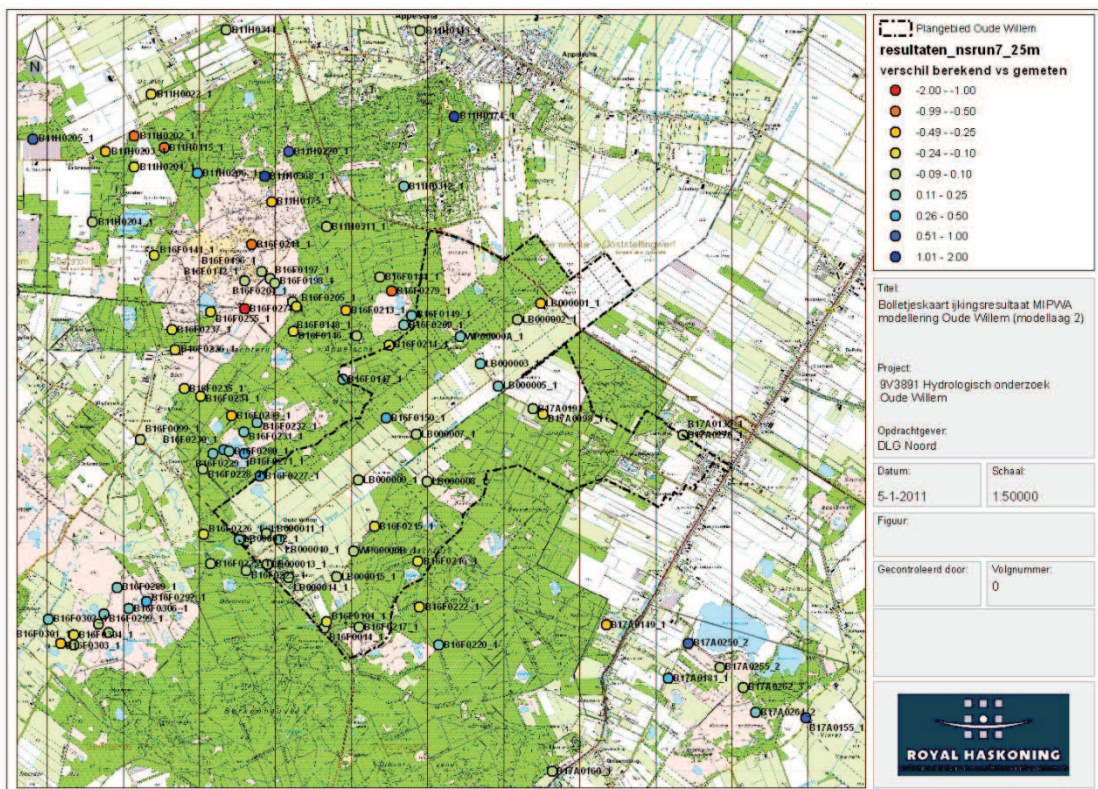
Figuur 9. Bolletjeskaart ijkingsresultaat modellaag 2 (berekende standen t.o.v. gemeten standen)
