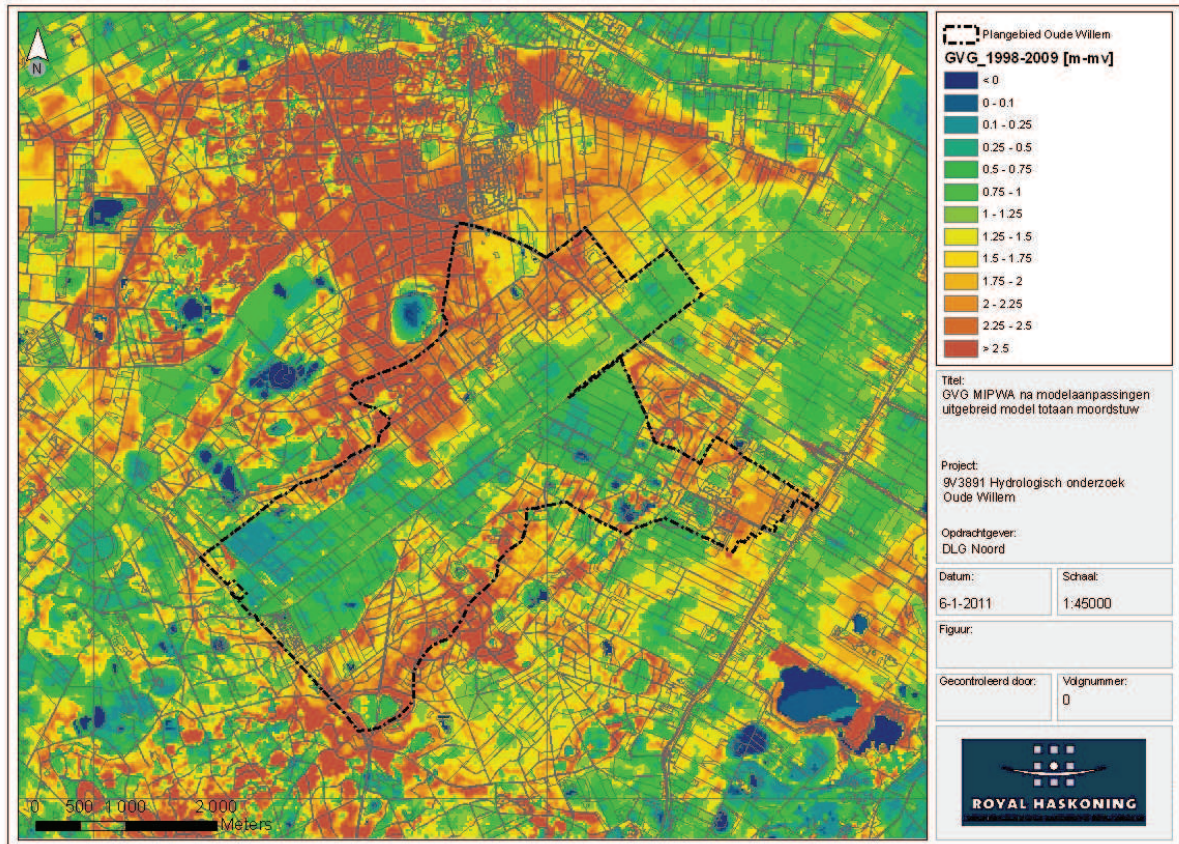
Figuur 14. GVG na modelaanpassingen
