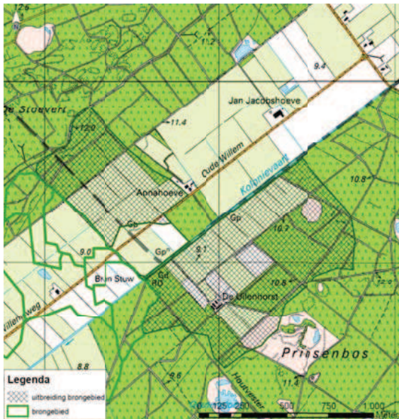
Figuur 19. Begrenzing brongebied Oude Willem m.b.t. afwatering richting Moordstuw
