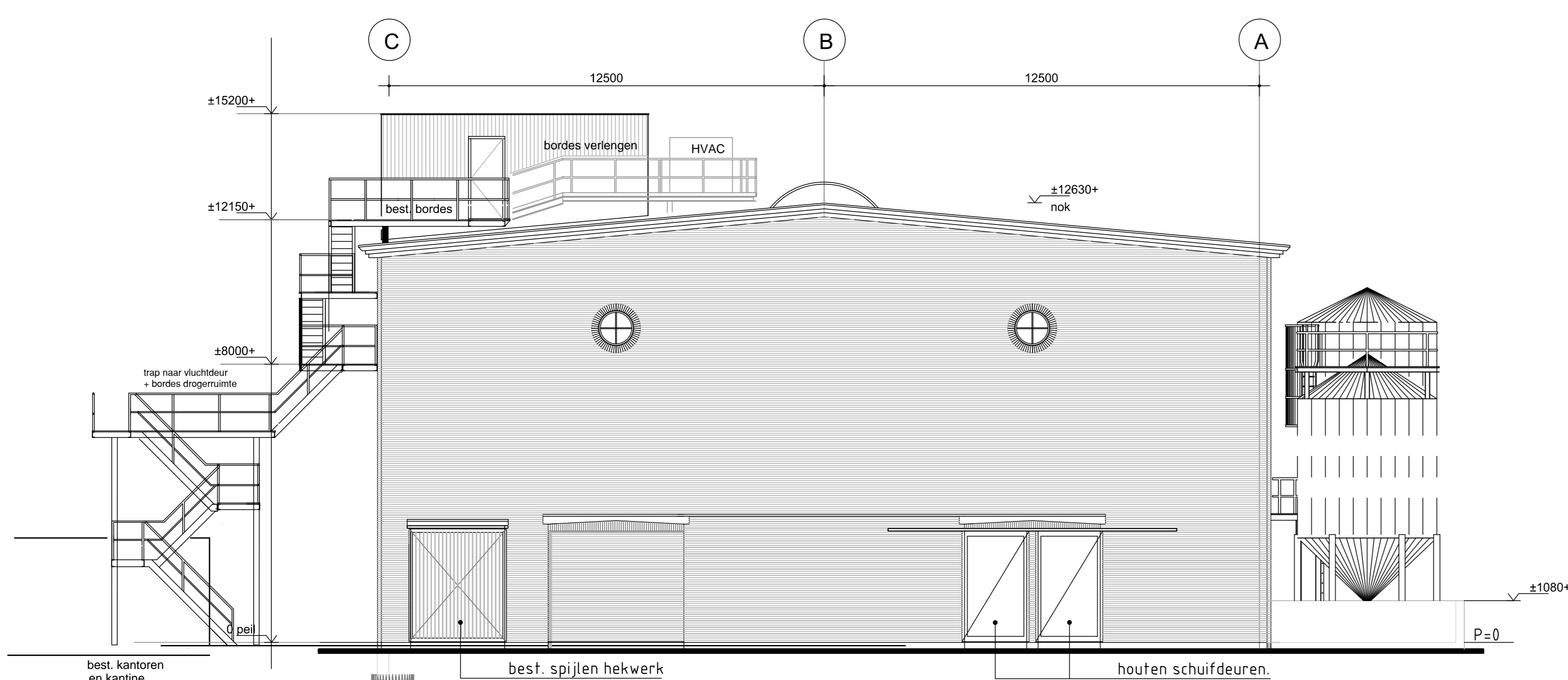
Rechter Zijaanzicht (Noordgevel) scale 1:100
