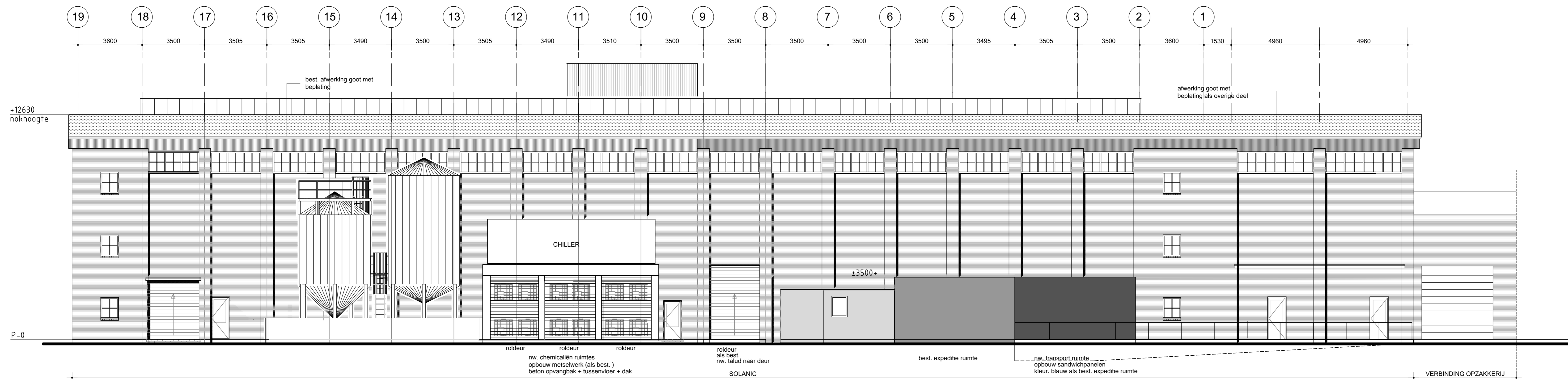
best. achteraanzicht (Westgevel) scale 1:100
