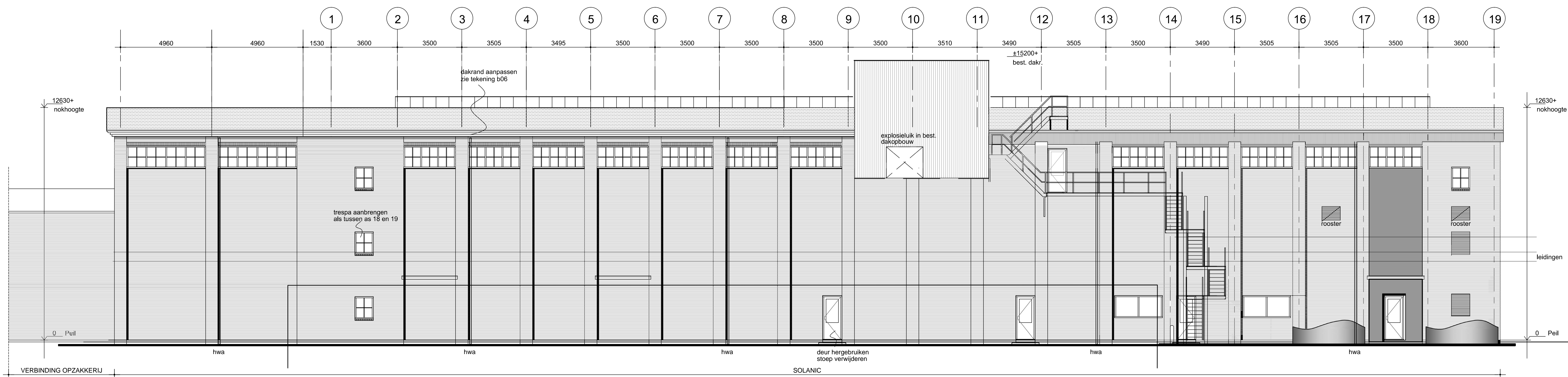
best. Vooraanzicht (Oostgevel) scale 1:100
